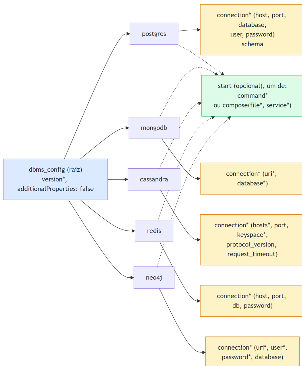
Figura 9 – Estrutura do JSON Schema de conexão (dbms_config).
