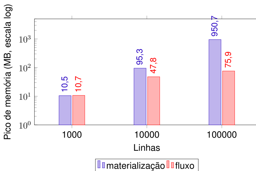
Figura 19 – Pico de memória por modelo de execução em função do volume (multifonte, escala logarítmica): a materialização cresce com o arquivo; o fluxo achata.
