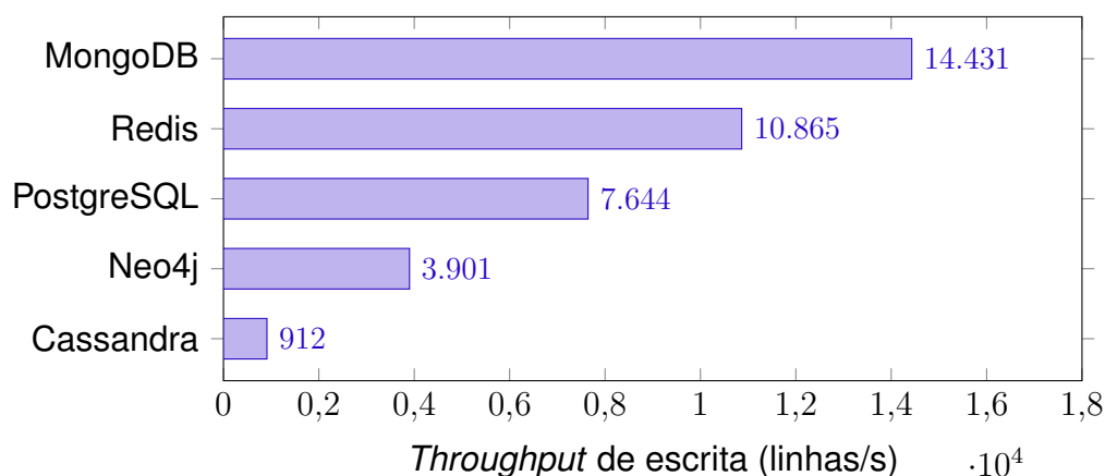
Figura 18 – Throughput de escrita por SGBD ( N = 100\,000 , multifonte, materialização, estratégia otimizada). Campanha sem instrumentação de memória.
