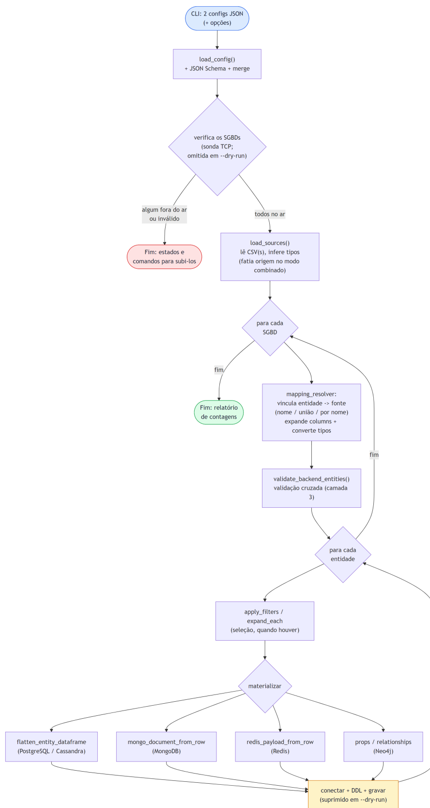
Figura 11 – Algoritmo de execução da importação PolyglotImportCSV.
