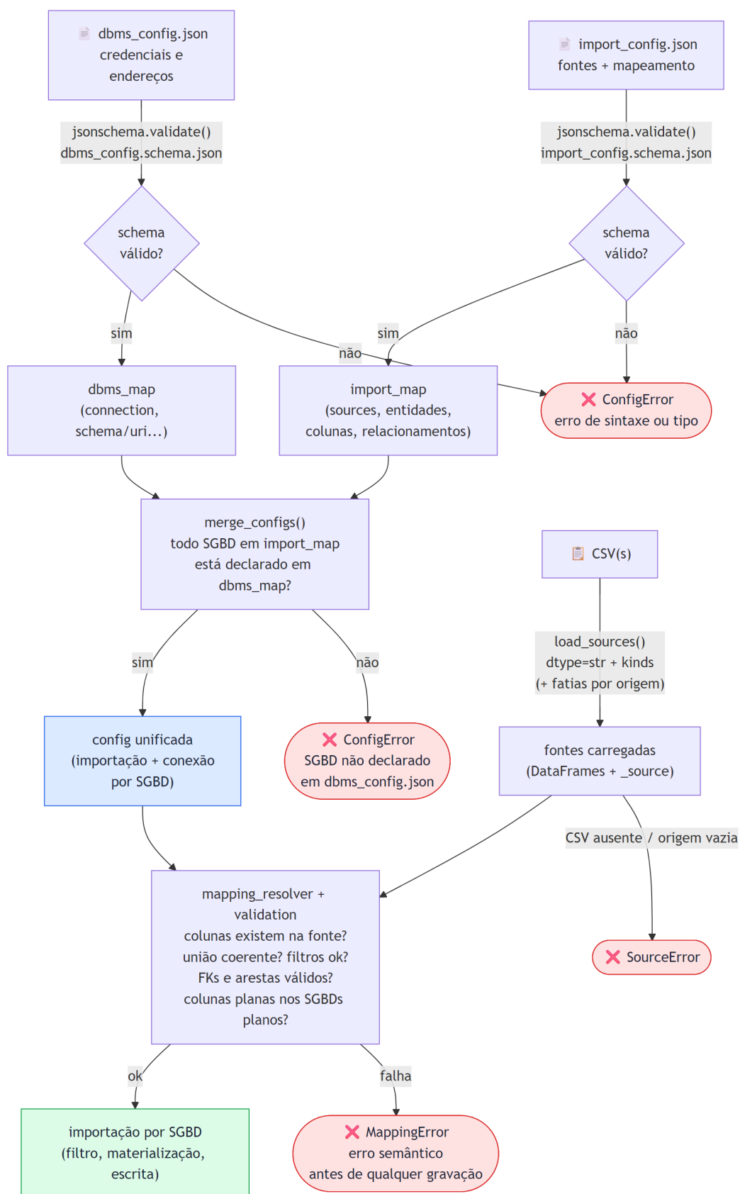
Figura 10 – Fluxo de carregamento e validação das entradas da ferramenta.
