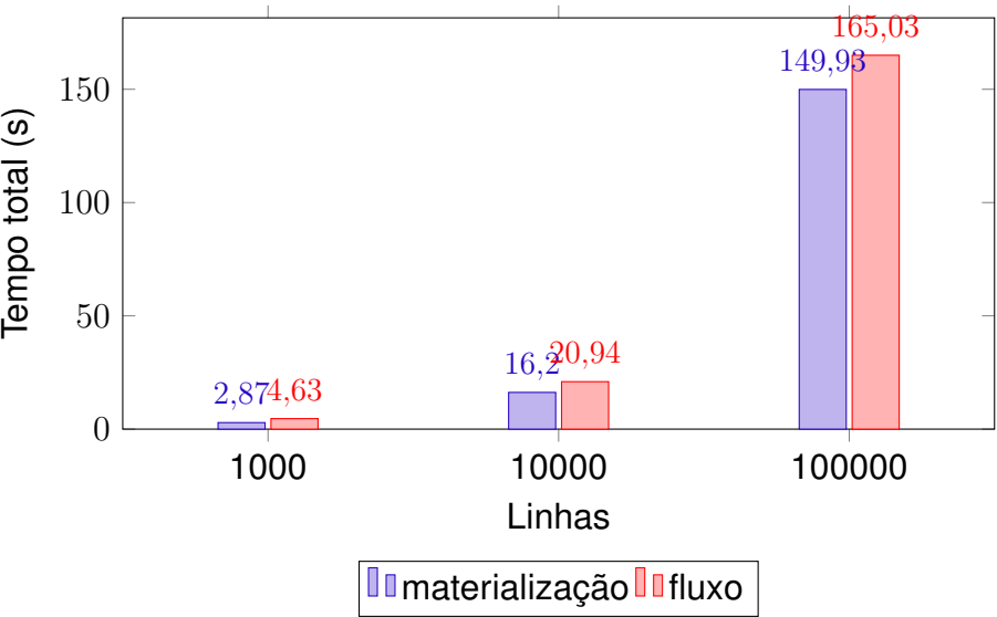
Figura 20 – Tempo total por modelo de execução em função do volume (multifonte): o sobrecusto do fluxo encolhe de +61% para +10% à medida que a escrita passa a dominar.
