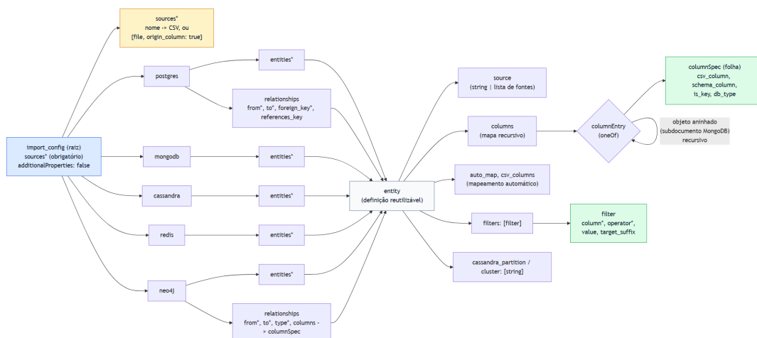
Figura 8 – Estrutura do JSON Schema de importação ( import_config ).
