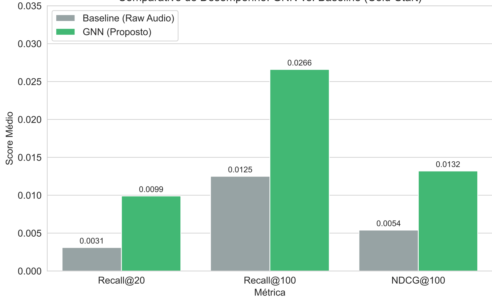
Comparativo de Desempenho: GNN vs. Baseline (Cold-Start)
