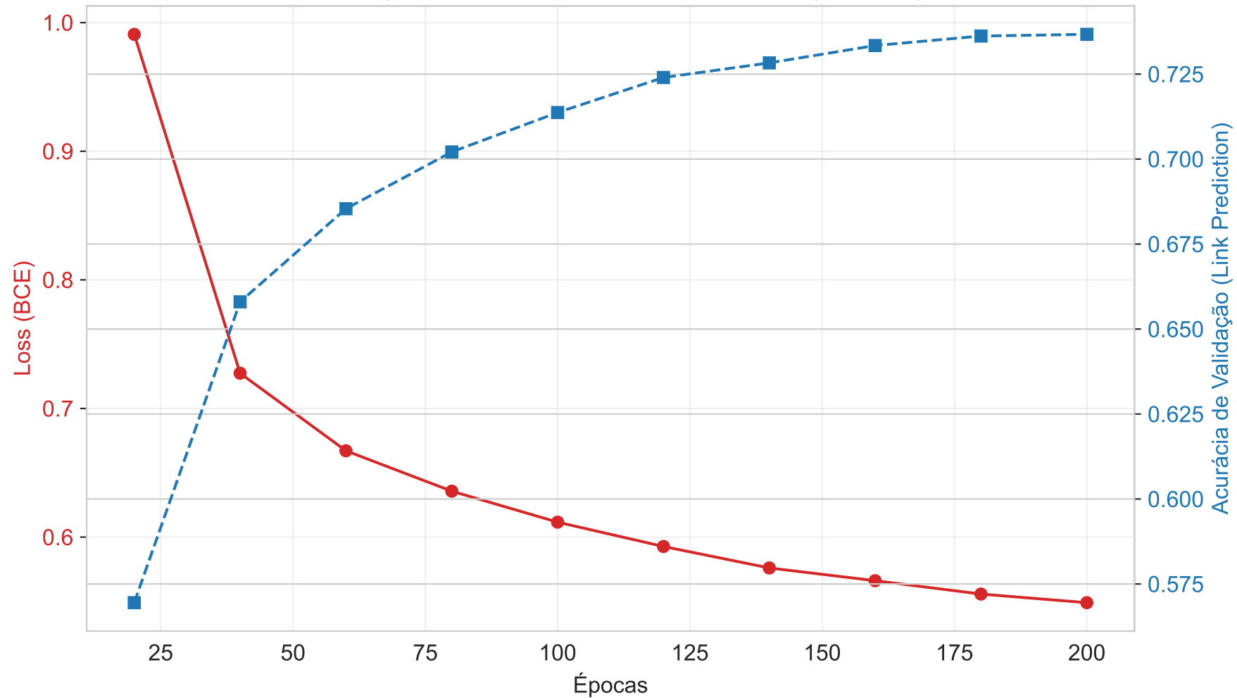
Convergência do Treinamento GraphSAGE (Seed 42)
