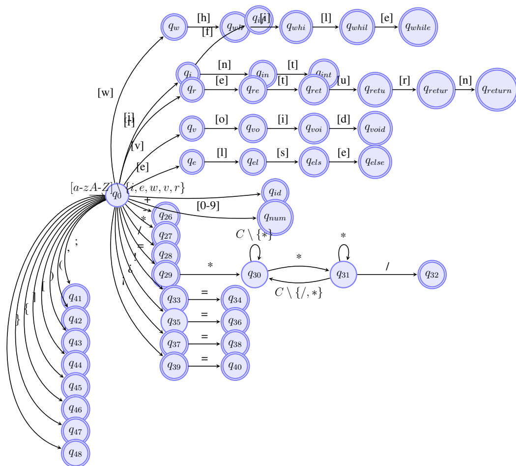
Figura 2. DFA minimizado final unificado com palavras-chave, operadores e símbolos especiais.
