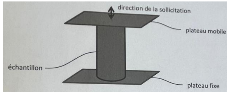
FIGURE 1 – Schéma de l'échantillon et direction de la sollicitation
