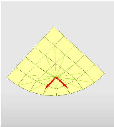
FIGURE 5 – Encastrement de la face inférieure.
