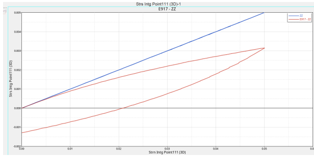
(a) \sigma = f(\epsilon) à la vitesse v_{min}
