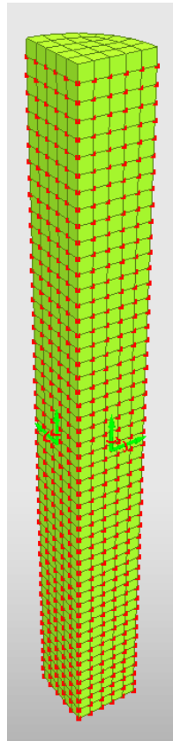
FIGURE 6 – Conditions de symétrie radiale.
