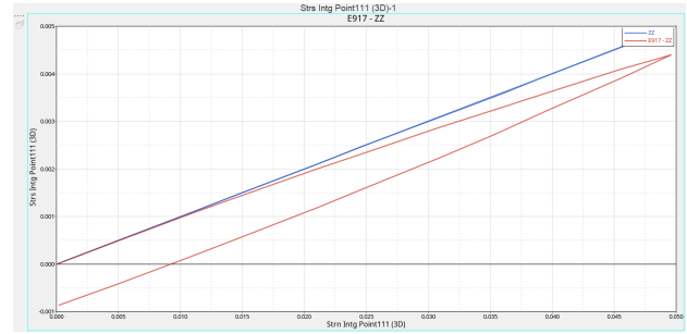
(b) \sigma = f(\epsilon) à la vitesse v_{max}
