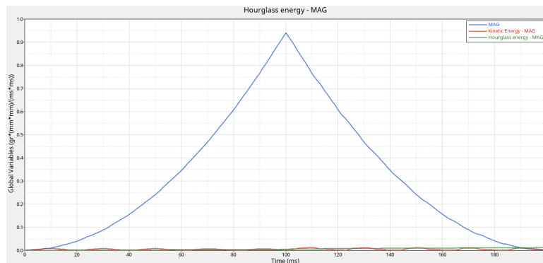
FIGURE 15 – Suivi des énergies (Interne, Cinétique et Hourglass)
