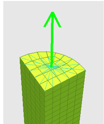
FIGURE 7 – Vitesse imposée (Face supérieure).
