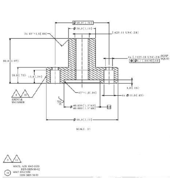
FIGURE 26 – P10 de l'outillage 956A8403G02
