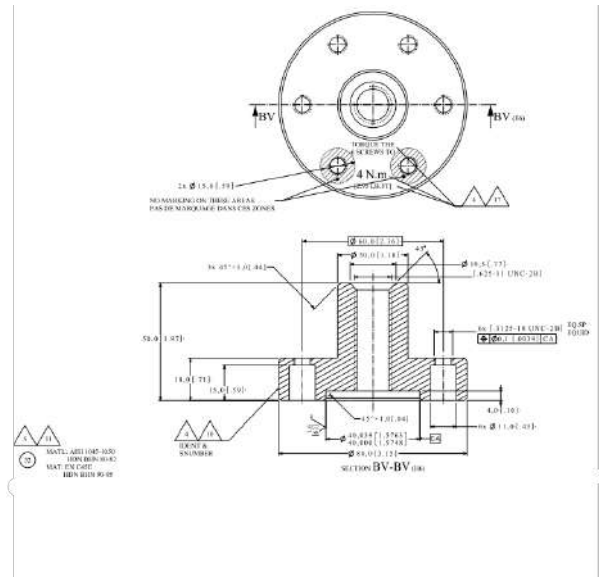
FIGURE 27 – P32 de l'outillage 956A8403G03
