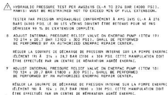
FIGURE 21 – Indication de test en pression
