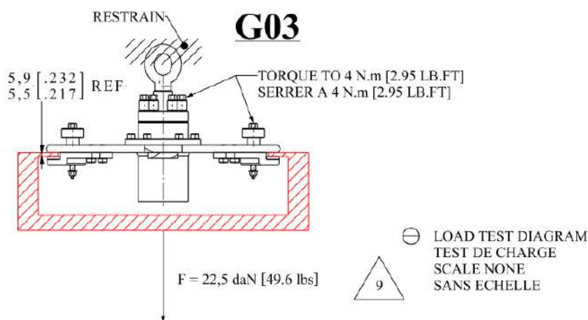
FIGURE 30 – Schéma du test en charge de l'outillage 956A8403G03
