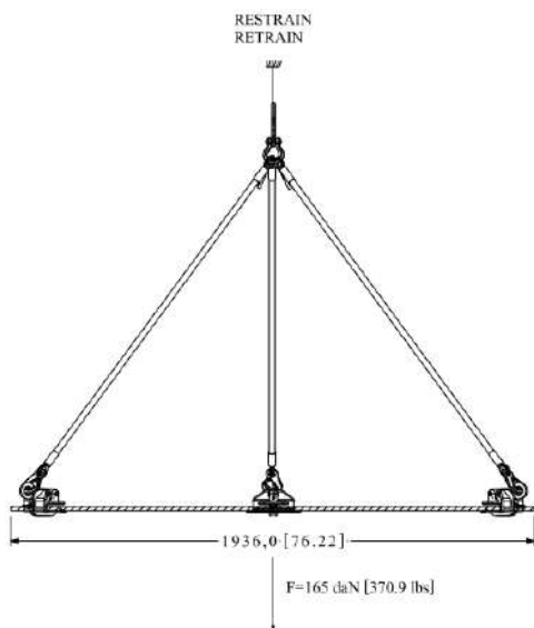
FIGURE 20 – Schéma d'un test en charge
