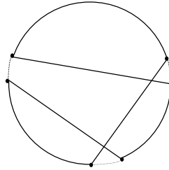
b) 3-Opt move
