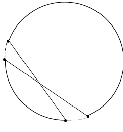
a) 2-Opt move
