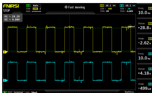
(A) Ensayo de la entrada digital.
