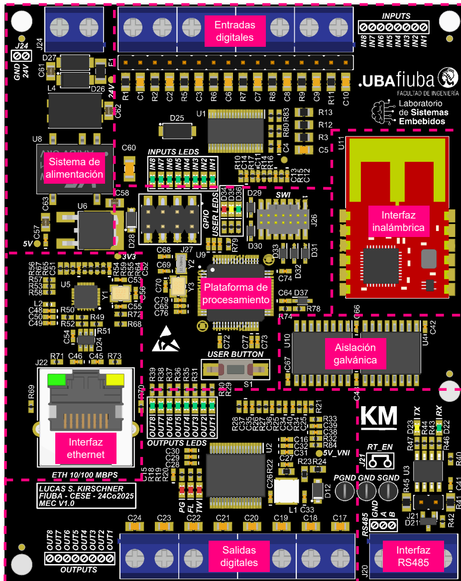
FIGURA 3.6. Vista tridimensional del PCB desarrollado.
