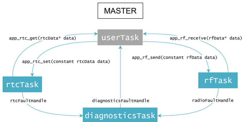
FIGURA 3.7. Organización general del firmware de la estación central.
