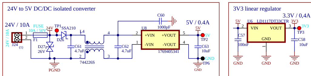
FIGURA 3.5. Esquema eléctrico de la etapa de alimentación.
