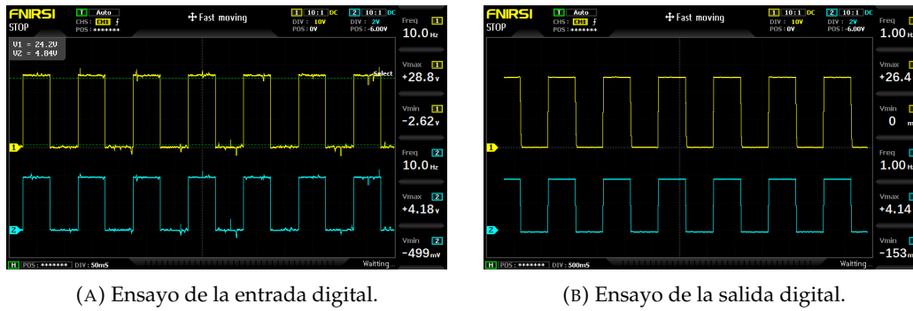
FIGURA 4.2. Señales registradas durante los ensayos de las etapas de entradas y salidas digitales.
