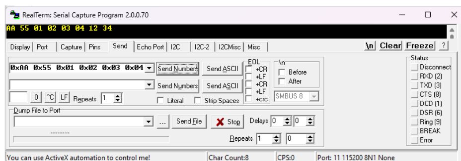
(A) Trama retransmitida visualizada mediante RealTerm.
