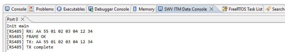
(B) Registro de recepción, validación y retransmisión mediante SWO.
