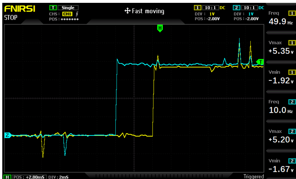
FIGURA 4.5. Medición de la latencia de comunicación inalámbrica entre la estación remota y la estación central mediante osciloscopio.
