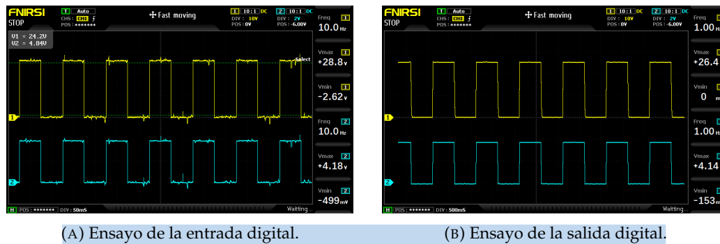
FIGURA 4.2. Señales registradas durante los ensayos de las etapas de entradas y salidas digitales.
