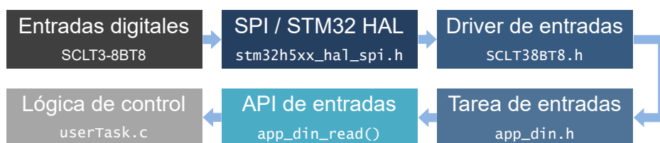
FIGURA 3.9. Integración hardware-software de las entradas digitales.
