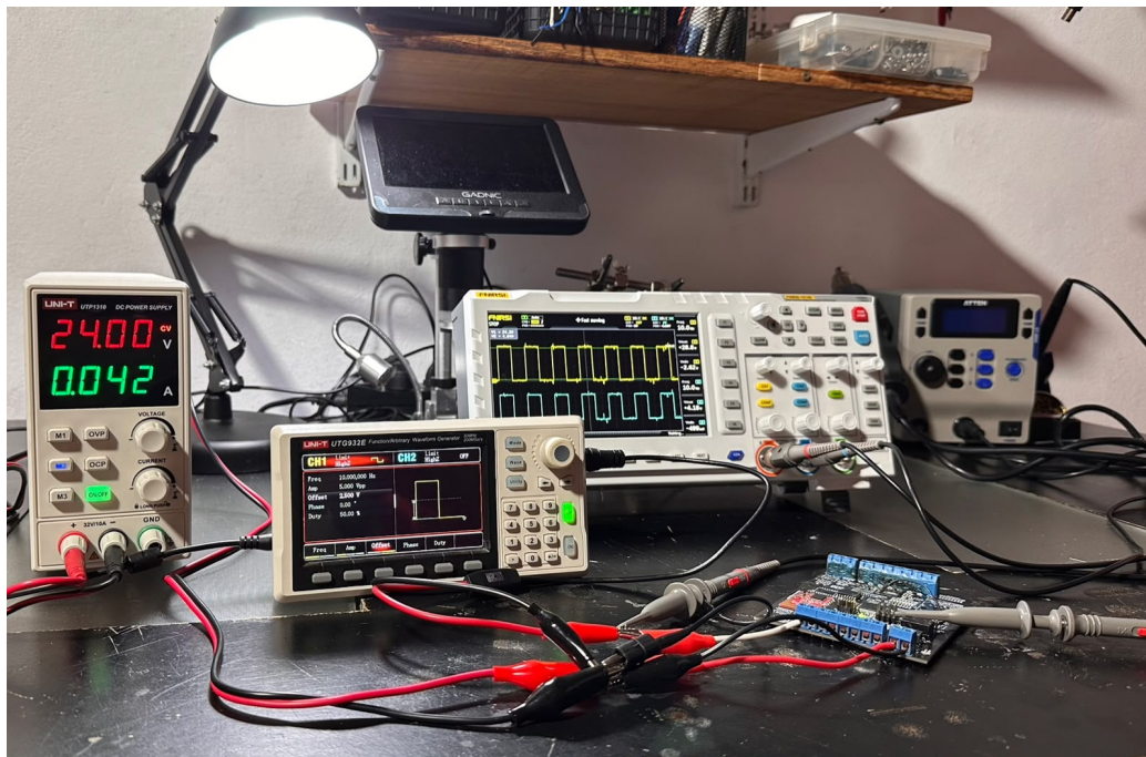
FIGURA 4.1. Banco de trabajo e instrumental utilizado para la realización de los ensayos.
