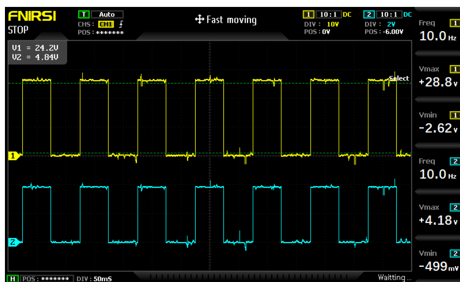
FIGURA 4.2. Señal aplicada a la entrada digital 1 y estado correspondiente replicado sobre el pin GPIO0.
