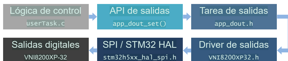
FIGURA 3.10. Integración hardware-software de las salidas digitales.
