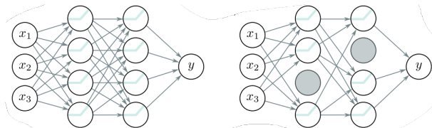
Esquerda: rede densa. Direita: rede com unidades desligadas.
