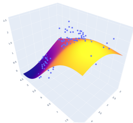
Figura: SVM
