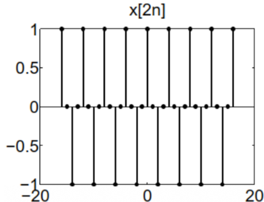
Sinal comprimido
