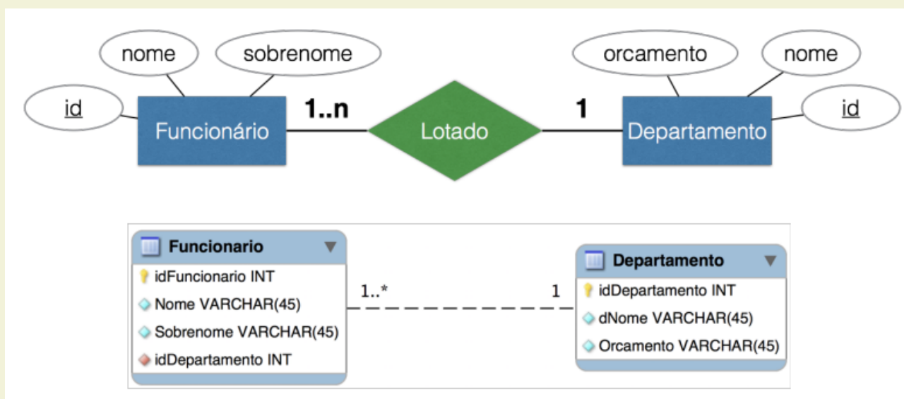
Figura 1: Esquema de banco de dados com as relações Funcionario e Departamento
