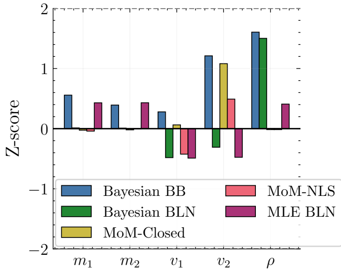
Moment PPCs
