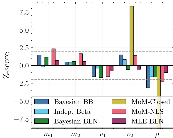
Moment PPCs
