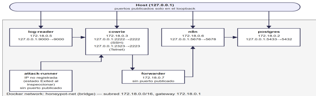
Figura 5.1: Diagrama de contenedores Docker con puertos y red, con las direcciones asignadas por Docker en el lote L0 (subred 172.18.0.0/16). La subred fue 172.19.0.0/16 en W1 y W2 y 172.18.0.0/16 en C1. En las tres el simulador se ejecutó desde attack-runner (§5.2.2). Fuente: Elaboración propia.
