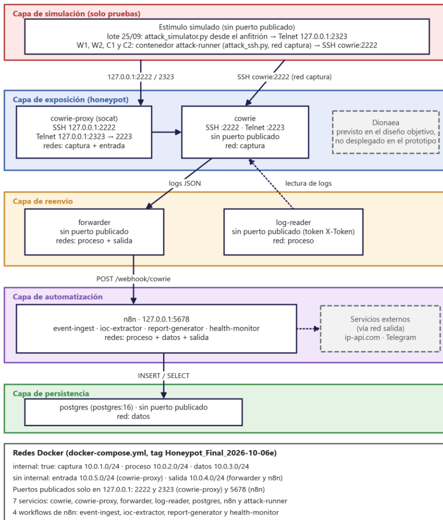
Figura 4.1: Arquitectura general de la solución por capas, en la configuración final. Dionaea figura con línea punteada como componente previsto en el diseño objetivo, no desplegado (§5.2.1). En esta configuración log-reader y postgres no publican puertos, Cowrie publica los suyos mediante cowrie-proxy, n8n ejecuta cuatro workflows (incluido health-monitor) y las redes Docker son captura, proceso y datos (internal) más entrada y salida (Tabla 5.2, §5.2.2). El simulador atacó por Telnet (puerto 2323) en el lote L0 y por SSH (puerto 2222) en las validaciones W1, W2, C1, C2 y C3. Fuente: Elaboración propia.
