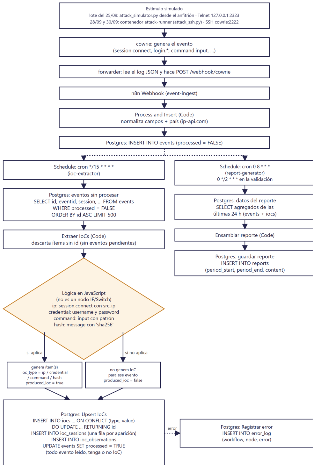
Figura I-2: Flujo de datos desde la captura del evento hasta la generación del reporte, con el extractor vigente en la validación del 30/09/2026 (filtro de ítems vacíos, registro en ioc_sessions y rama de error hacia error_log ). Fuente: Elaboración propia.
