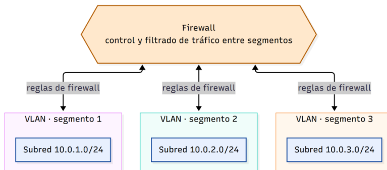
Figura 4.2: Topología de red con segmentación VLAN y reglas de firewall — diseño objetivo. El prototipo no implementa VLAN ni firewall: las validaciones L0 a C1 usaron una red Docker única; desde el 05/10/2026 (validación C2) sus tres capas se implementan con redes Docker (10.0.1.0/24, 10.0.2.0/24 y 10.0.3.0/24, rangos privados; Rekhter et al., 1996), con la red de datos como internal, y desde el 06/10/2026 las tres son internal, más una red de entrada y otra de salida (§5.2.2). Fuente: Elaboración propia.
