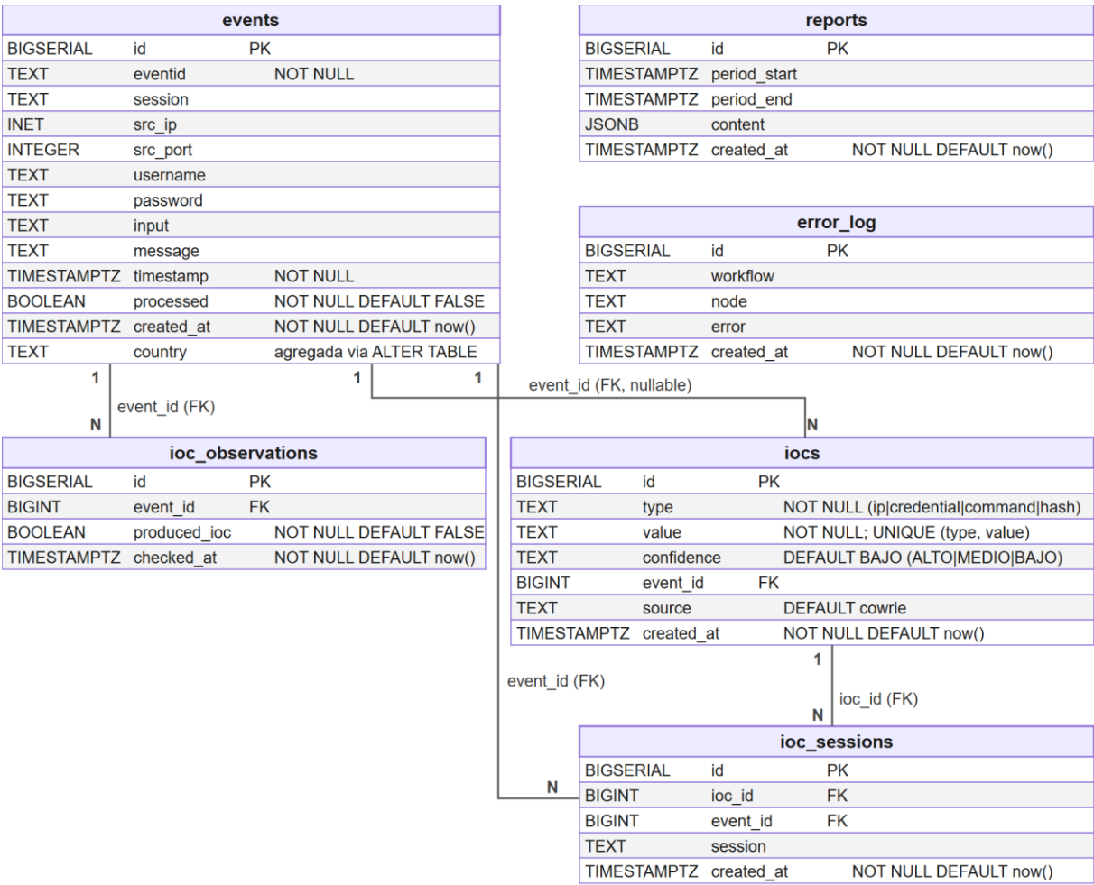
Figura III-1: Modelo de datos del prototipo (seis tablas de PostgreSQL definidas en db/schema.sql). Fuente: Elaboración propia.
