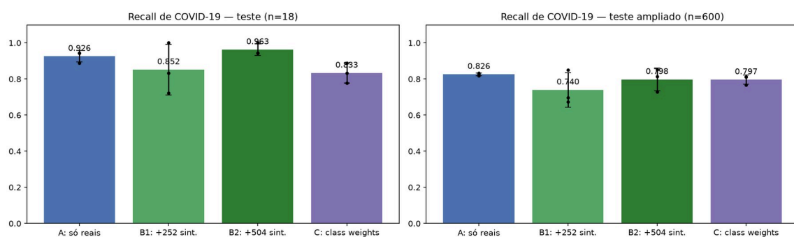
Recall de COVID-19 por condição (barras: média; pontos: sementes).
