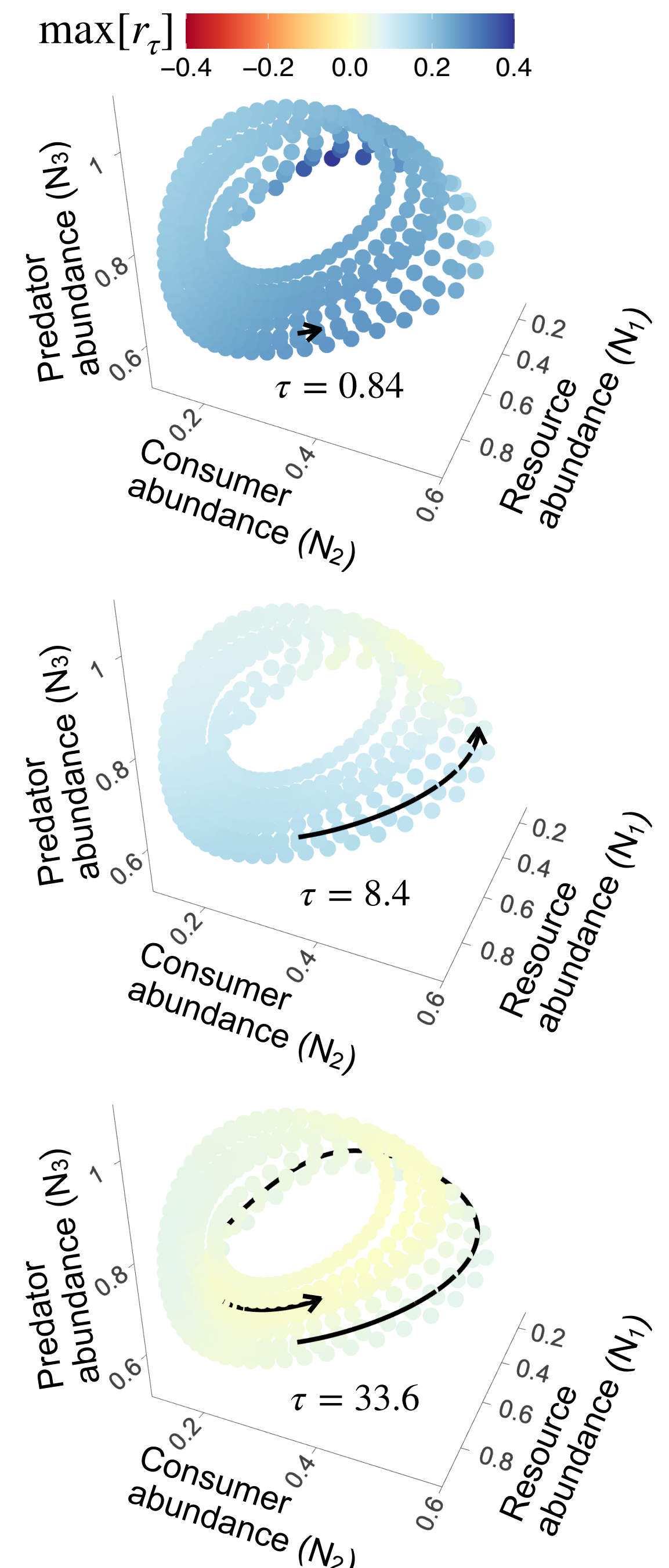
(d) 3-species chaotic attractor
