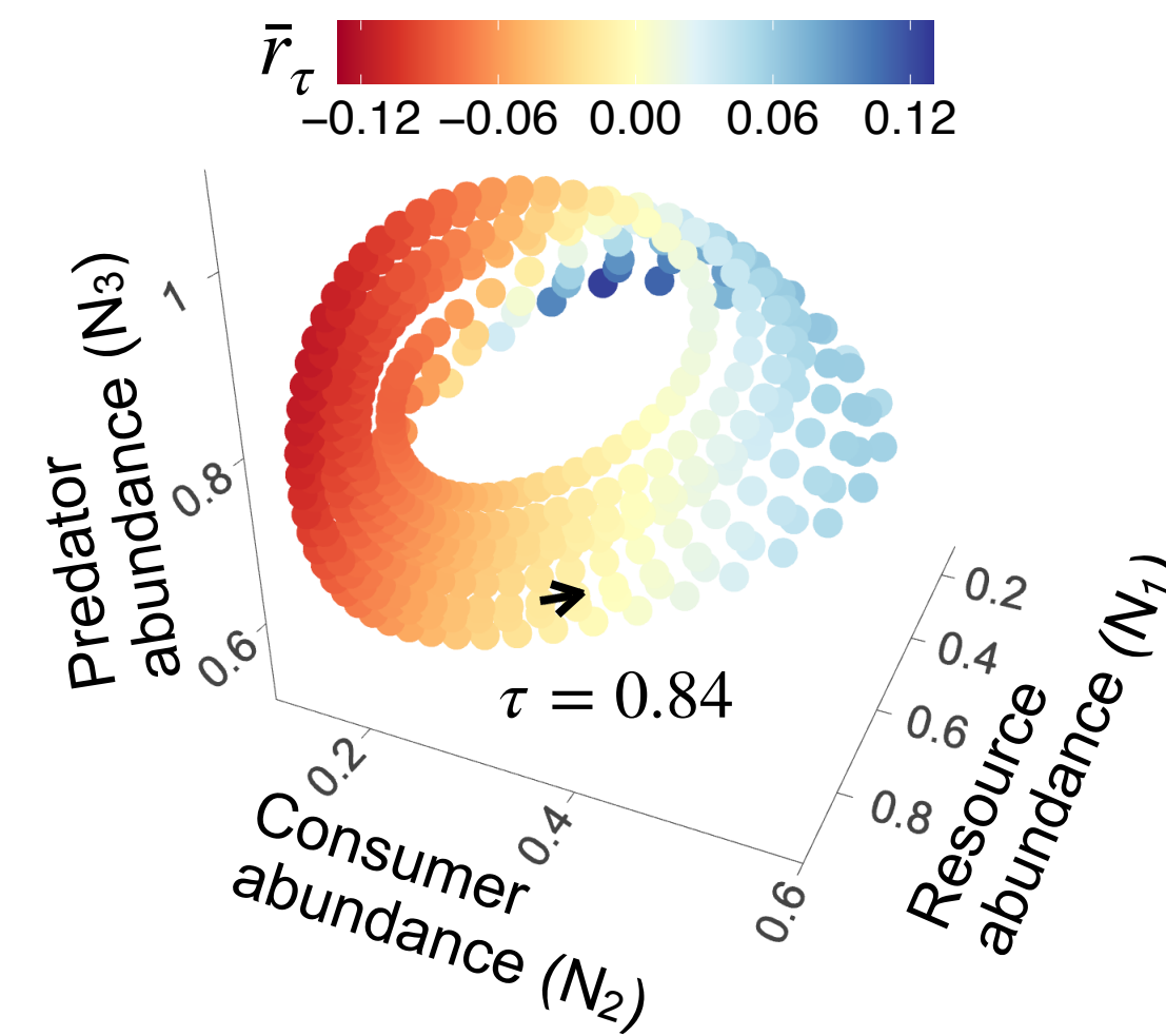
(d) 3-species chaotic attractor
