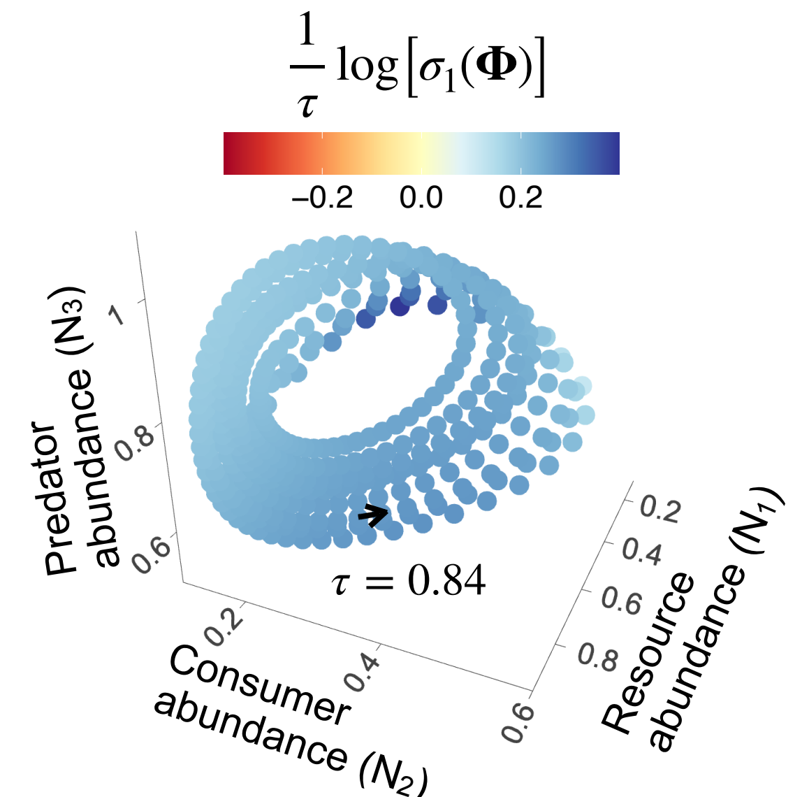
(d) 3-species chaotic attractor
