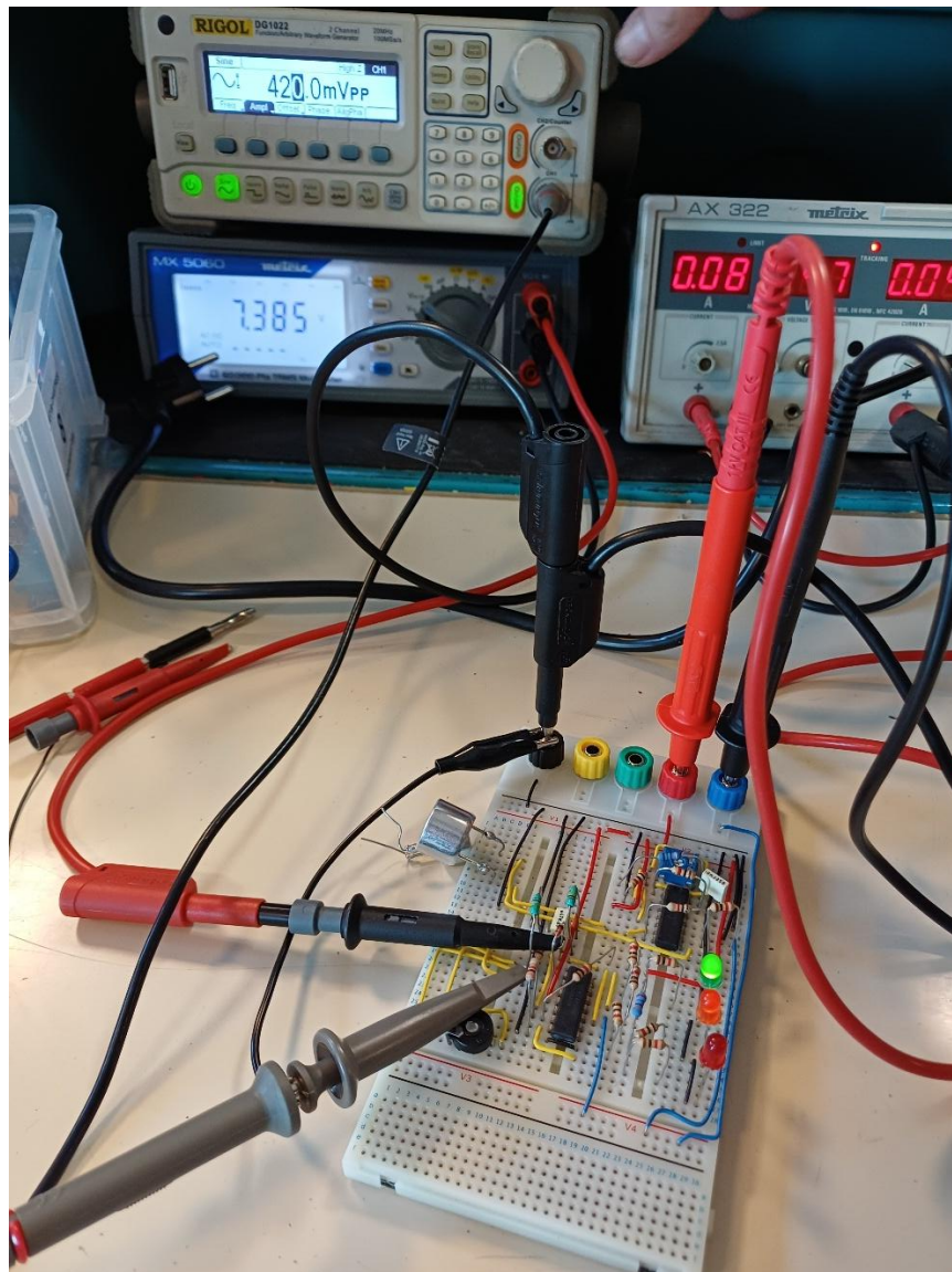
Uniquement LED verte allumée à 7,38 V.
