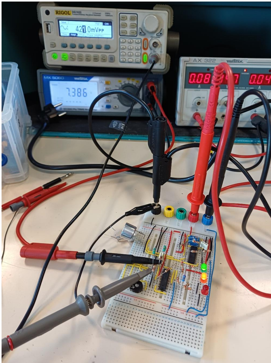
LEDs verte et orange allumées à partir de \approx 7,39 V.
