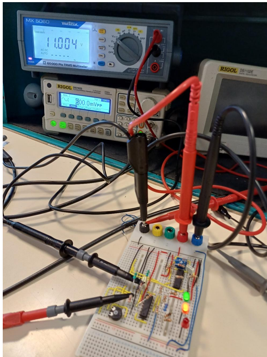
Uniquement LEDs verte et orange allumées à 11 V.
