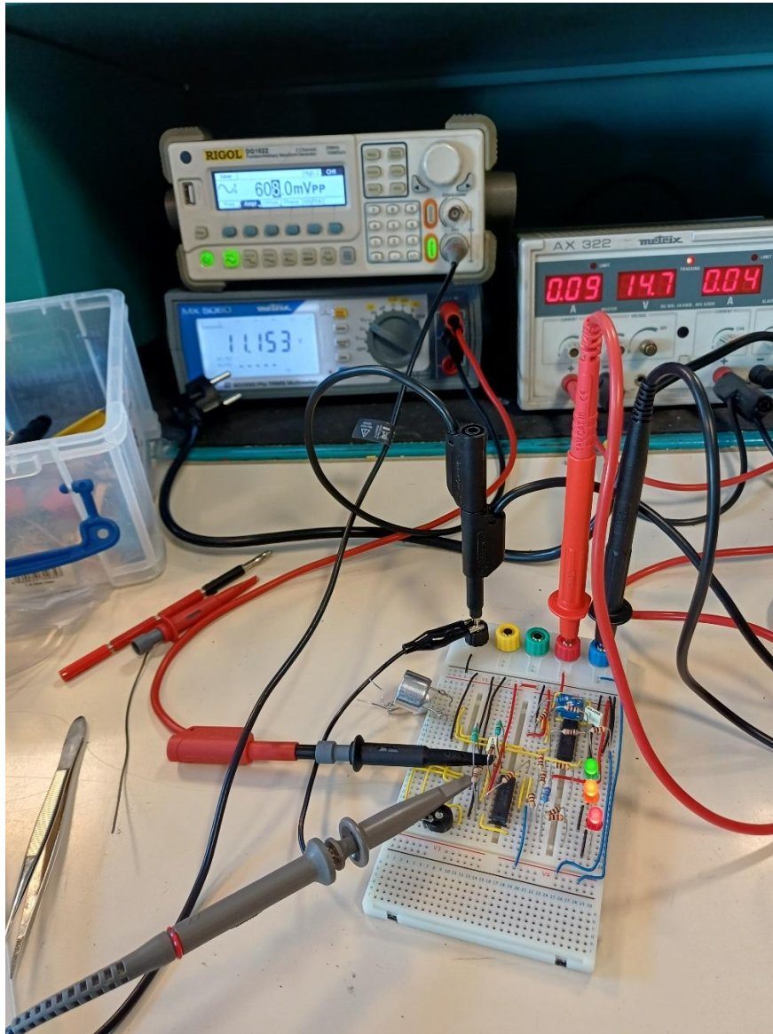
LEDs verte, orange et rouge allumées à partir de 11,15 V.
