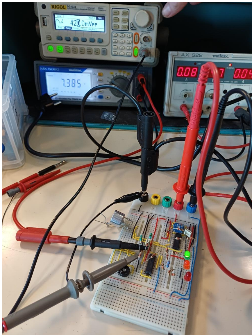
Uniquement LED verte allumée à 7,38 V.
