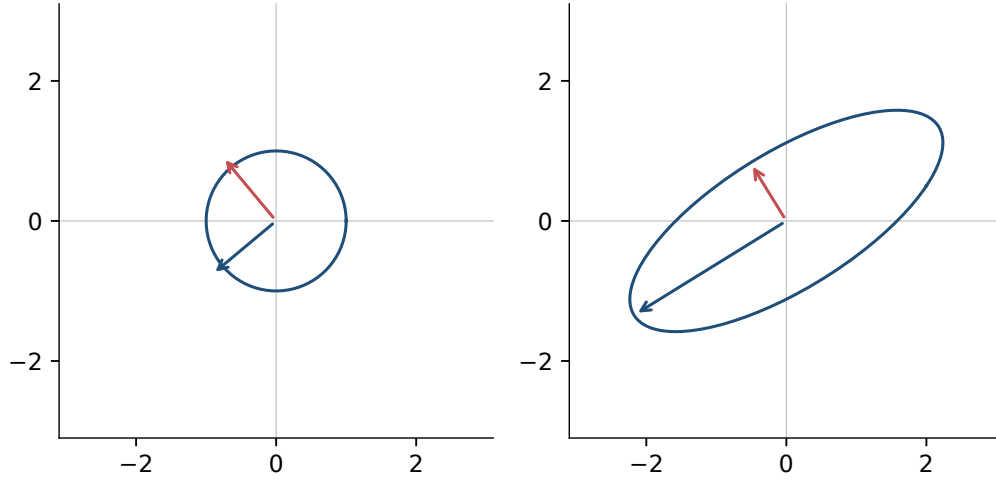
Figura 23: A transformação v \mapsto Av leva o círculo unitário em uma elipse. As setas à esquerda são as colunas de V ; à direita, os eixos \sigma_i u_i .
