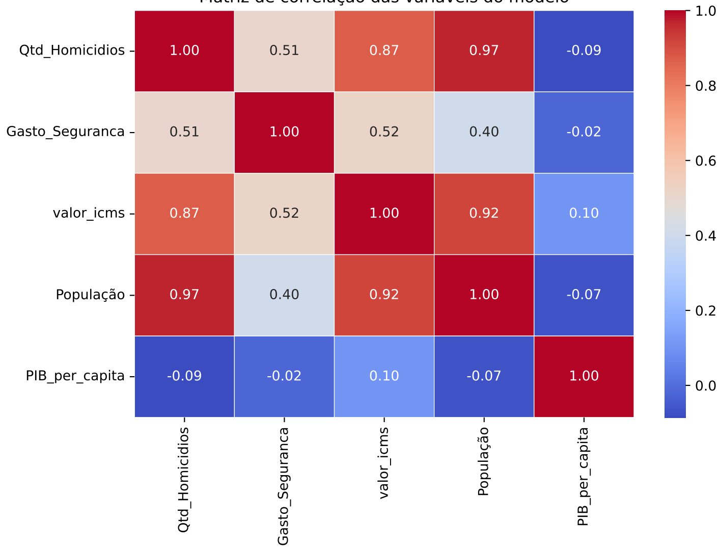
Matriz de correlação das variáveis do modelo
