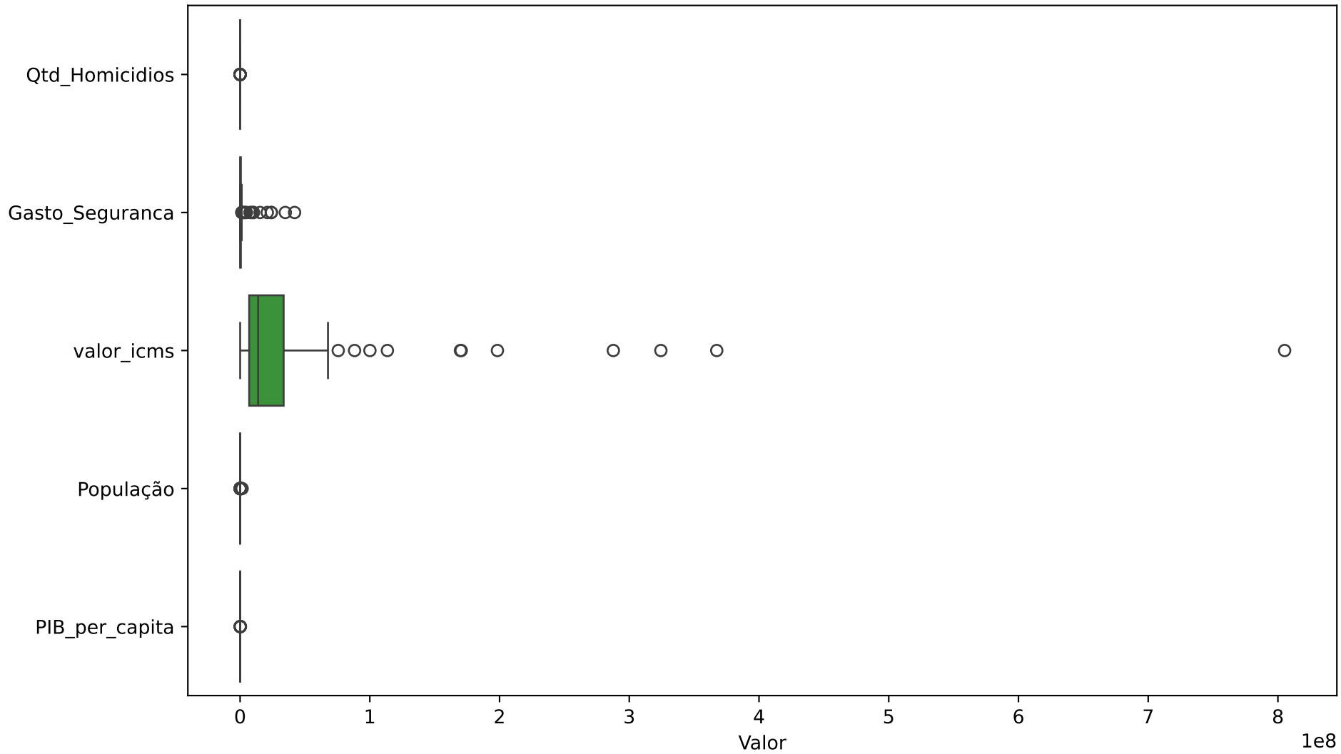
Boxplot das variáveis do modelo de regressão
