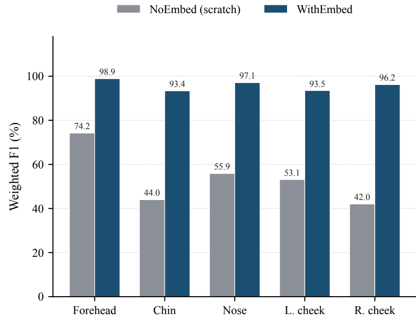
(a) Per-region weighted F1
