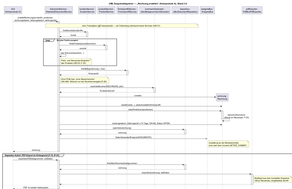
Abbildung 2: UML-Sequenzdiagramm „Rechnung erstellen“ (Komponente A)
