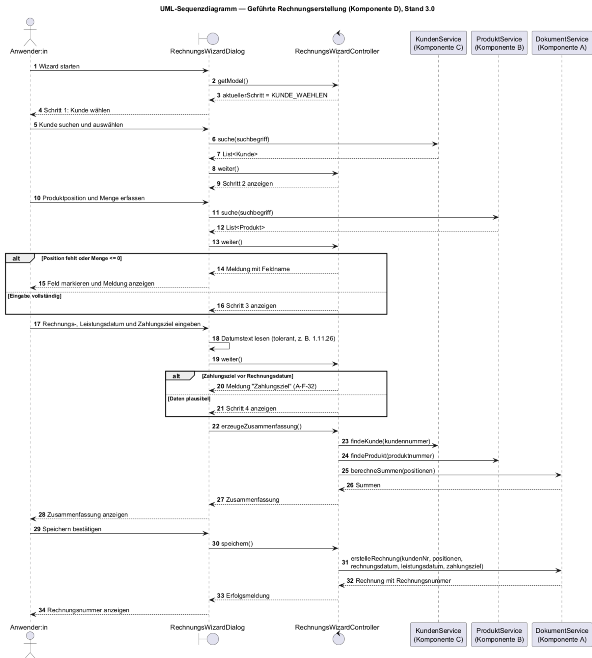
Abbildung 8: UML-Sequenzdiagramm Rechnungserstellung (Komponente D)
