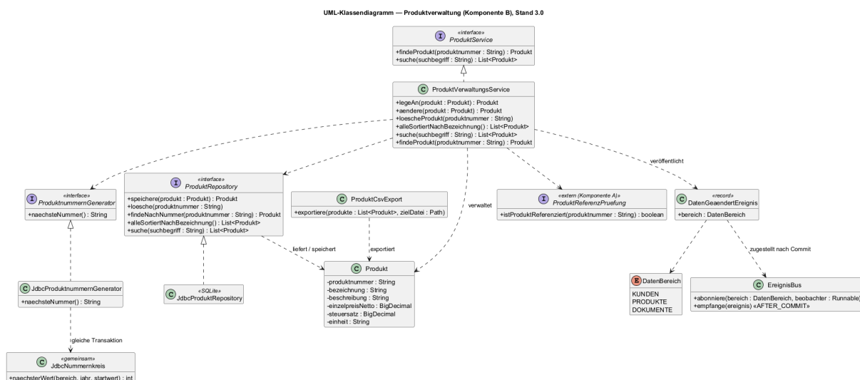
Abbildung 3: UML-Klassendiagramm Produktverwaltung (Komponente B)
