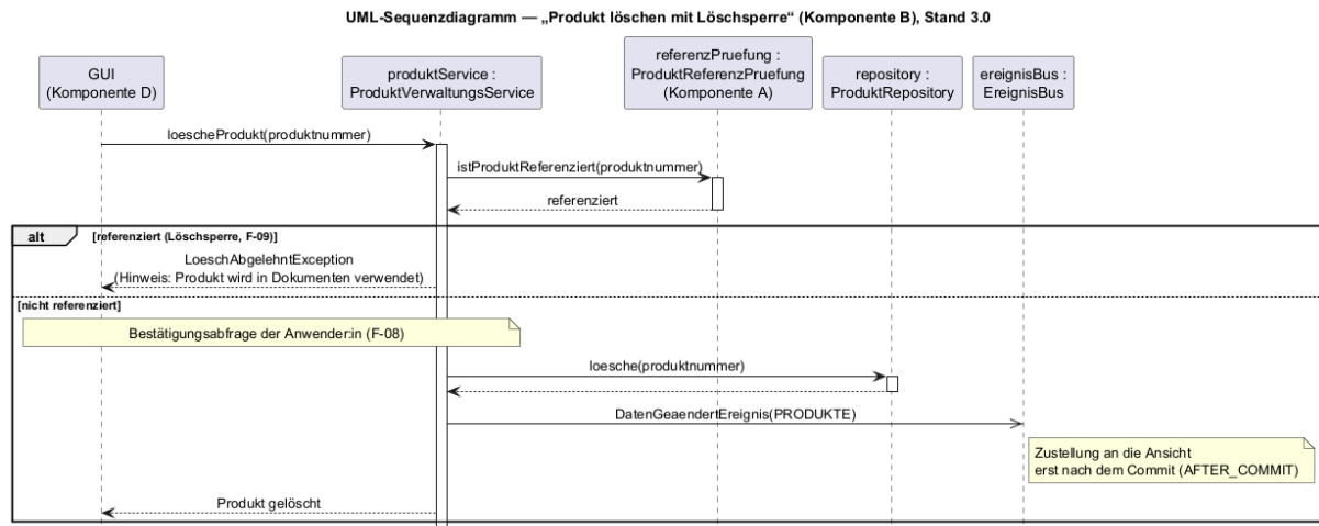
Abbildung 4: UML-Sequenzdiagramm „Produkt löschen mit Löchsperre“ (Komponente B)
