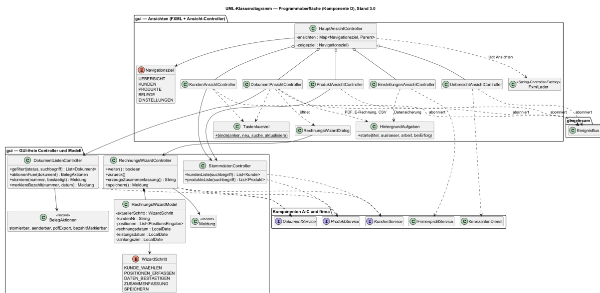
Abbildung 7: UML-Klassendiagramm Programmoberfläche (Komponente D)
