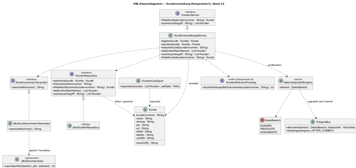
Abbildung 5: UML-Klassendiagramm Kundenverwaltung
