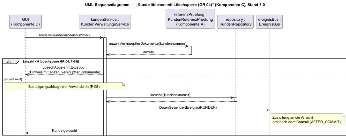
Abbildung 6: UML-Sequenzdiagramm „Kunde löschen mit Löchsperre (GR-04)“
