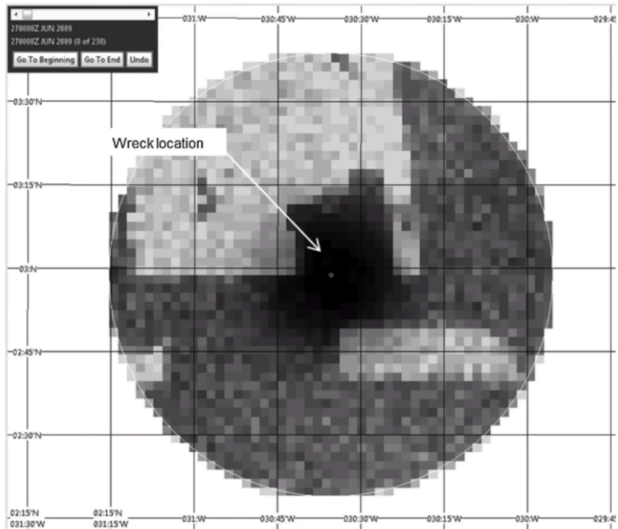
FIG. 7. Posterior distrubtion \tilde{P}_{1234} .
