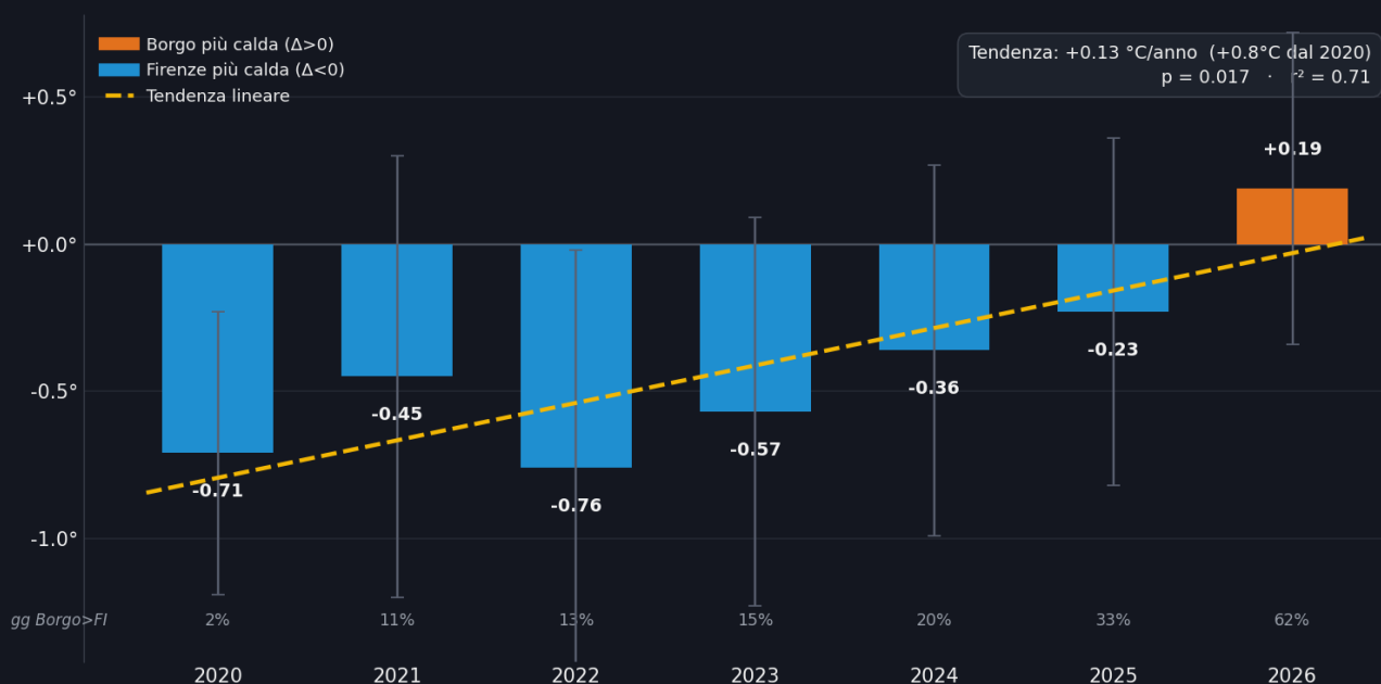
Fig. 4 — Scostamento medio estivo (giu–lug) delle Tmax, Borgo San Lorenzo – Firenze Università, 2020–2026. Barre di errore = deviazione standard giornaliera; sotto ogni anno la % di giorni con Borgo più calda.
