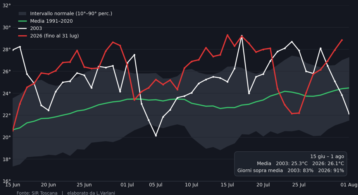
Fig. 1 — Temperatura media giornaliera 2003 e 2026 rispetto alla norma 1991-2020 (fascia grigia = 10°-90° percentile).
