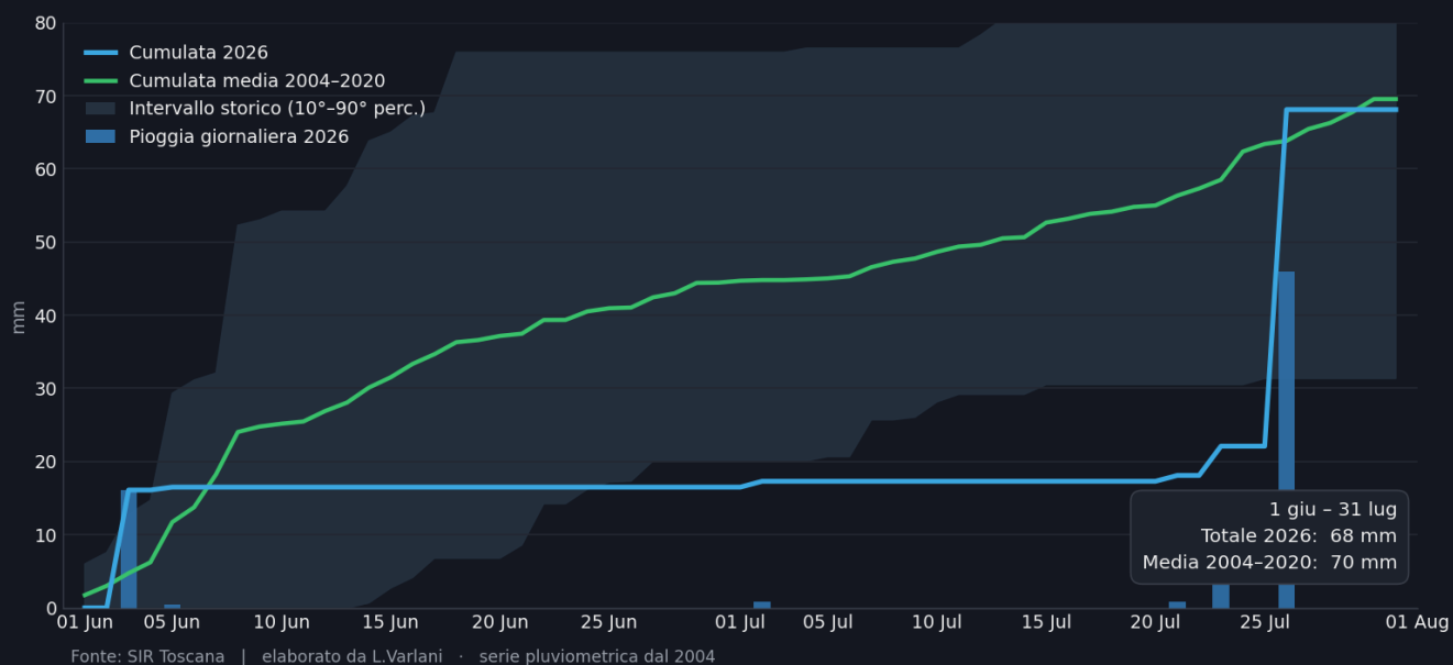
Fig. 3 — Pioggia giornaliera (barre) e cumulata 2026 vs media climatica 2004–2020 (giu–lug).
