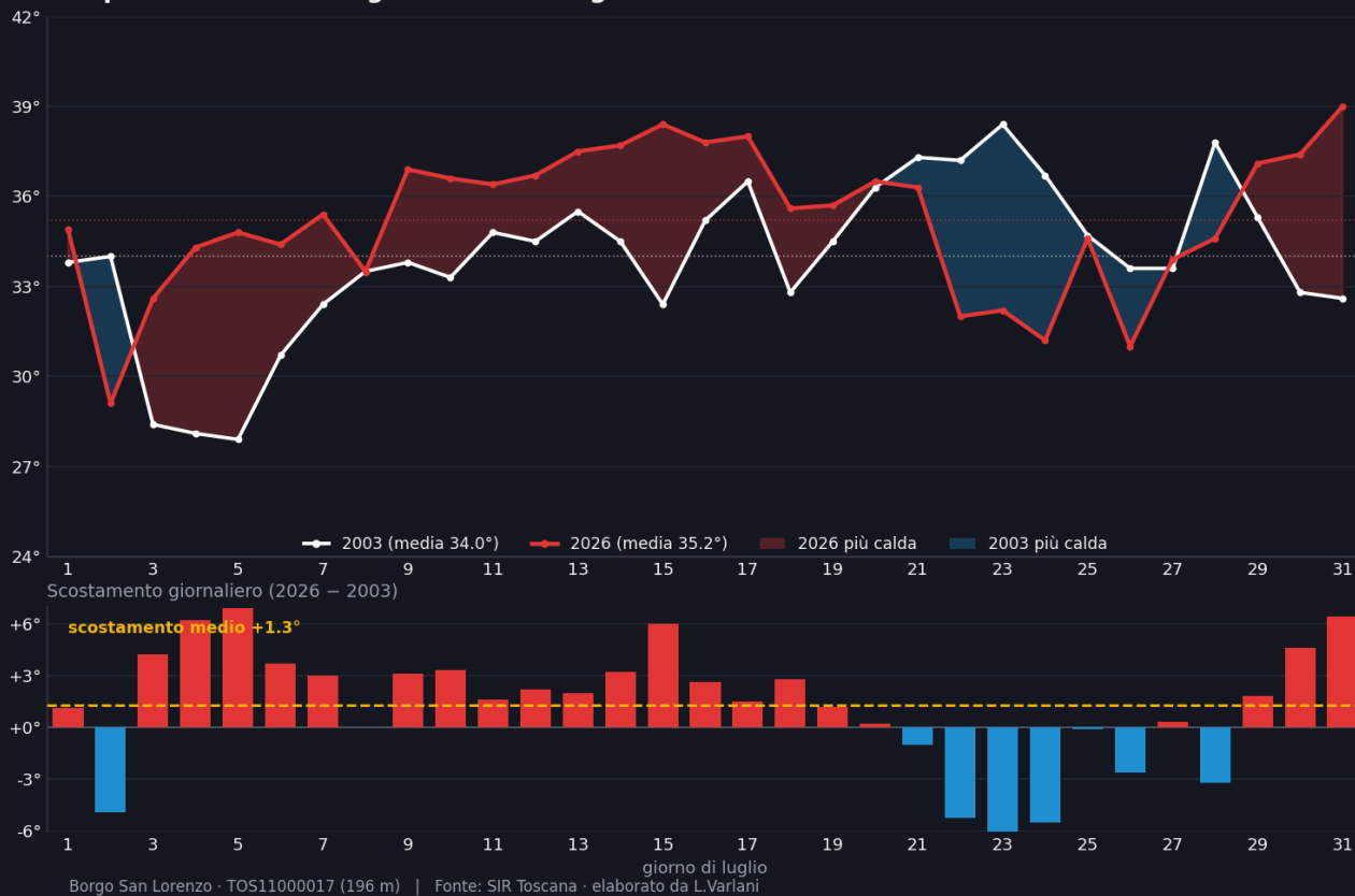
Temperature massime giornaliere di luglio: 2003 vs 2026
