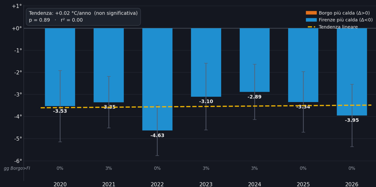
Fig. 5 — Scostamento medio estivo (giu-lug) delle Tmin, Borgo San Lorenzo – Firenze Università, 2020–2026. Valori sempre fortemente negativi e privi di tendenza.
