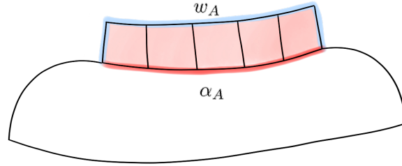
FIG. 21. Shortcut for an empty corridor w -arc A .
