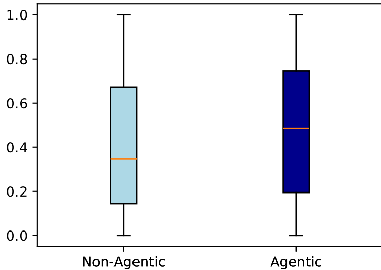
CodeBLEU
