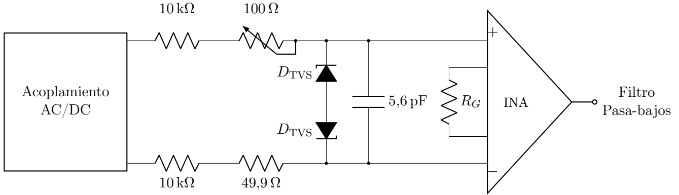
Figura 6: Amplificador de entrada.
