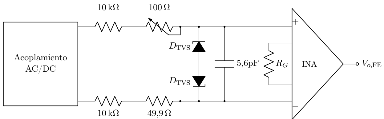
Figura 3: Amplificador de entrada.
