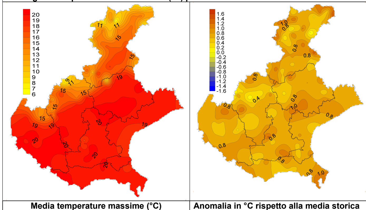
Fig. 2 - Temperatura massima anno (°C) periodo dicembre 2019 - novembre 2020
