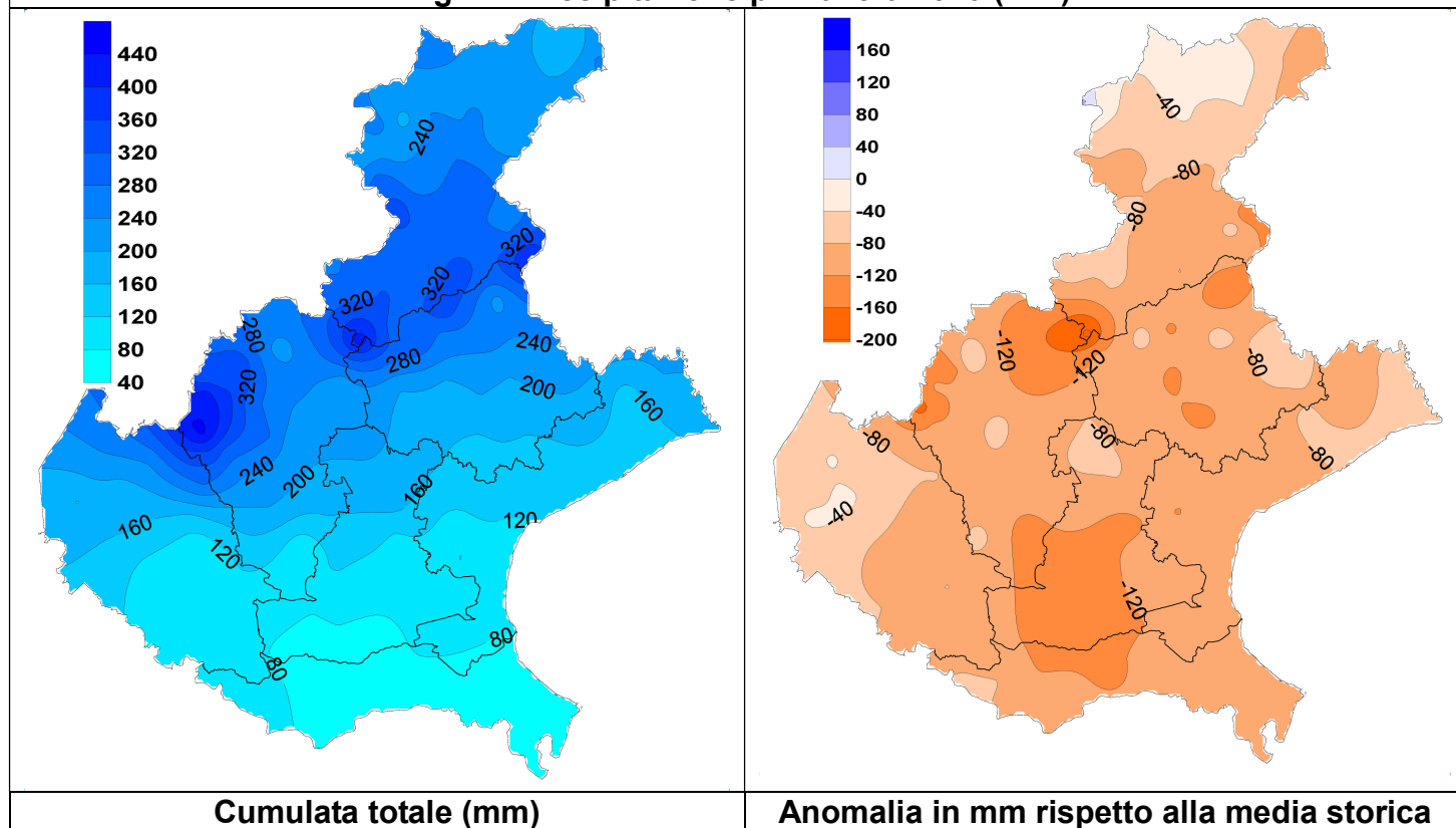
Fig. 4 – Precipitazione primavera 2020 (mm)
