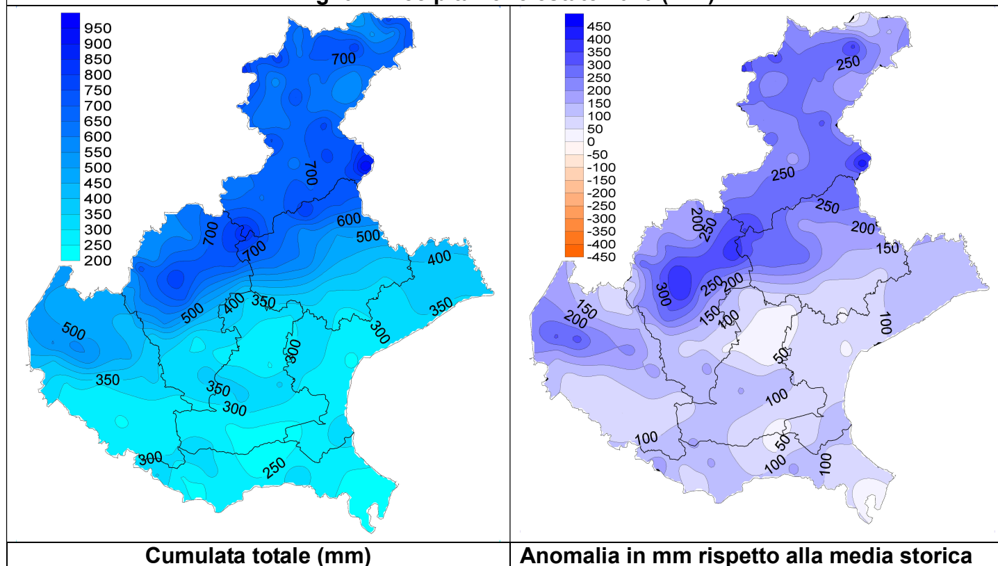
Fig. 6 – Precipitazione estate 2020 (mm)
