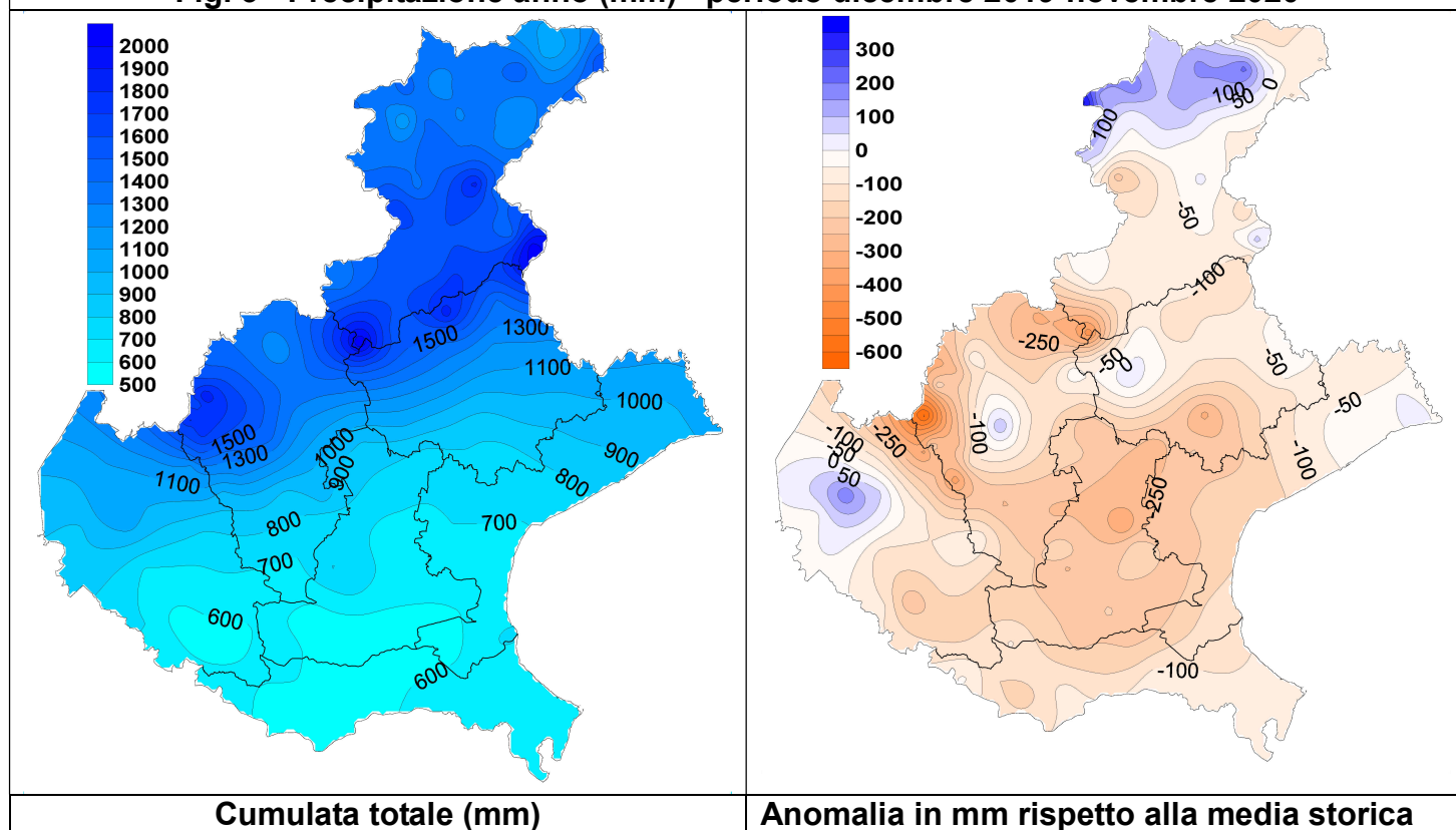
Fig. 3 - Precipitazione anno (mm) - periodo dicembre 2019-novembre 2020
