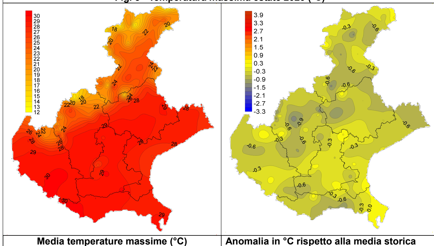
Fig. 5 - Temperatura massima estate 2020 (°C)
