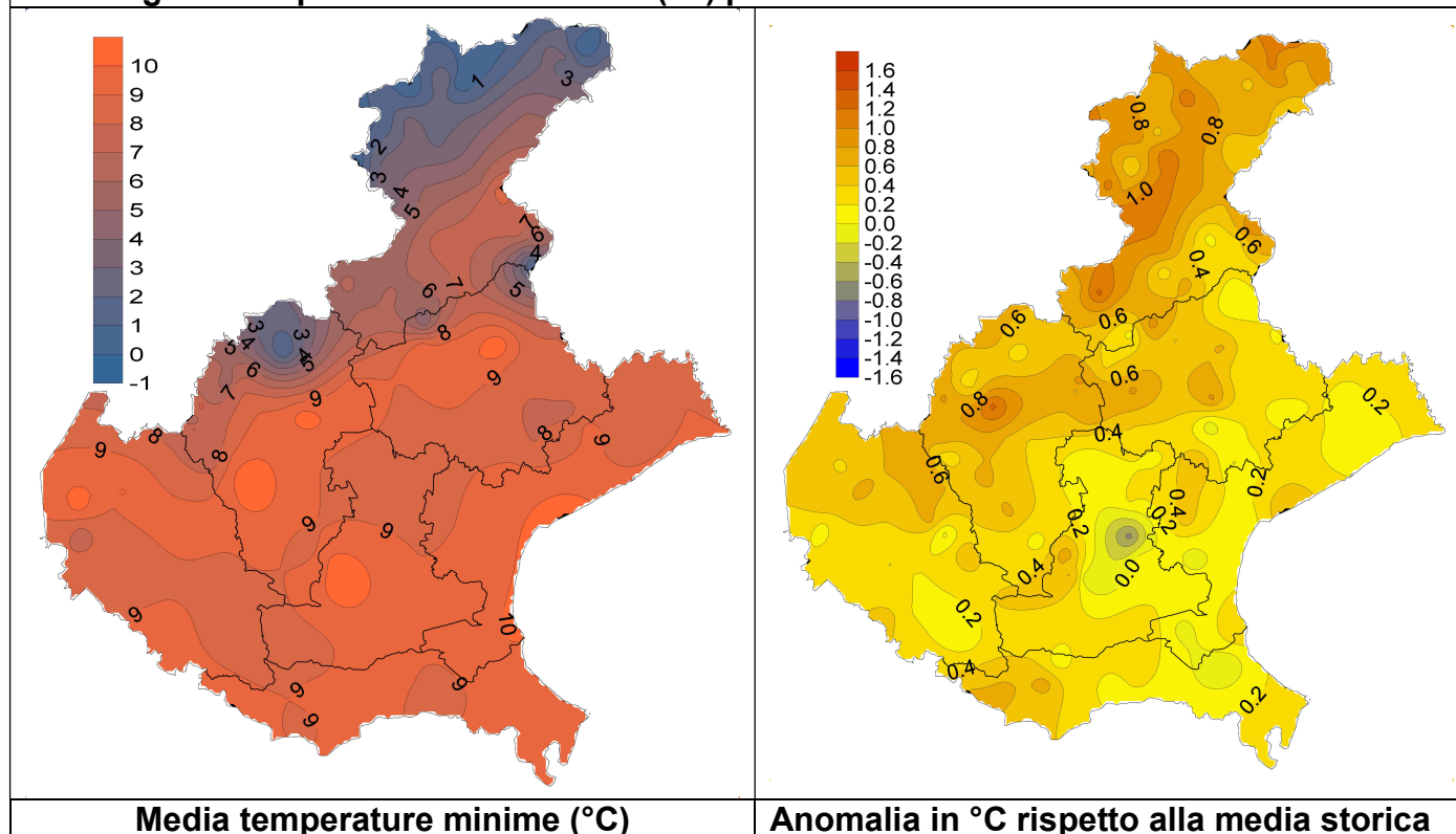
Fig. 1 - Temperatura minima anno (°C) periodo dicembre 2019 - novembre 2020
