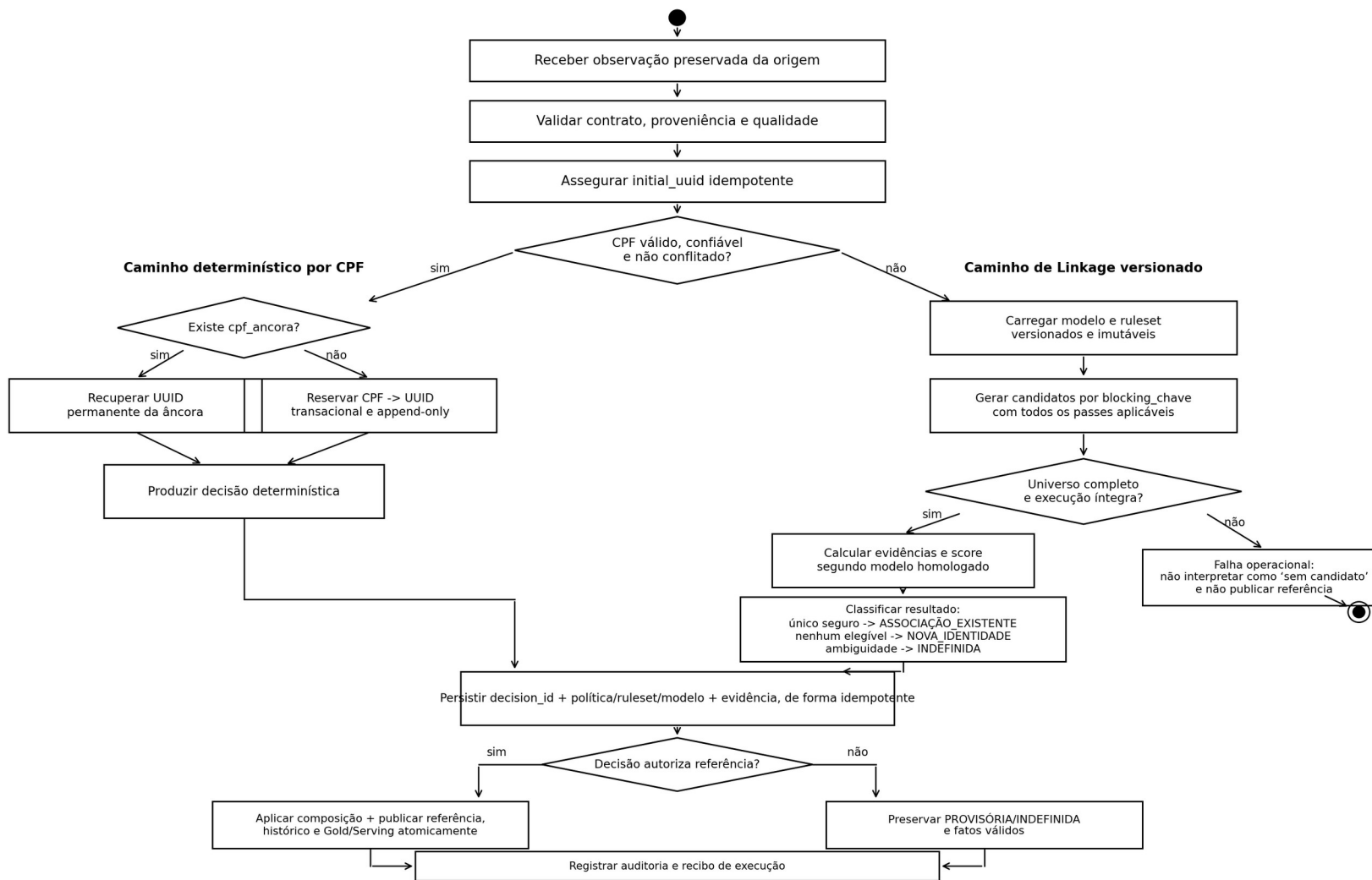
Figura 2 - Diagrama de atividade UML da resolução de identidade
