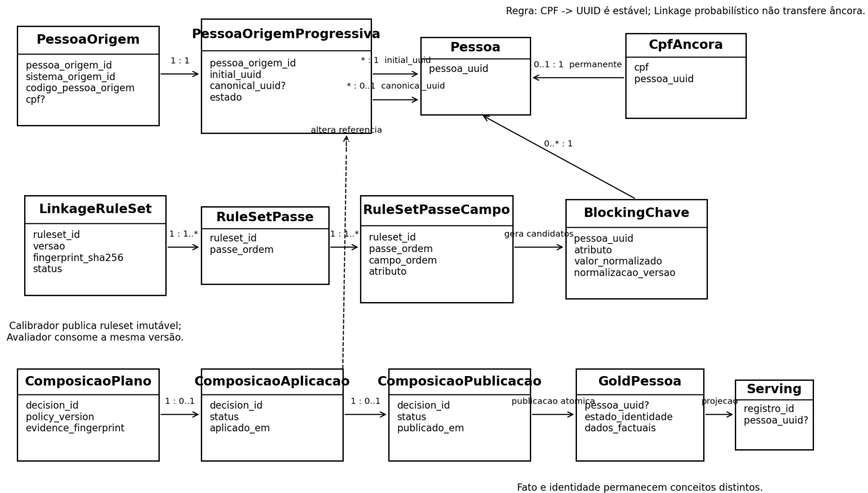
Figura 1 - Diagrama de classes UML da estrutura de Identidade/Linkage
