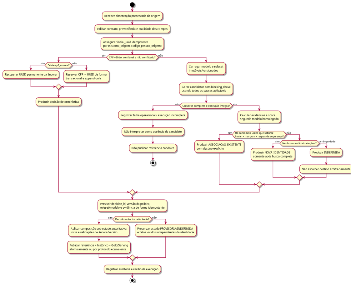
Figura 2 - Diagrama de atividade UML da resolução de identidade
