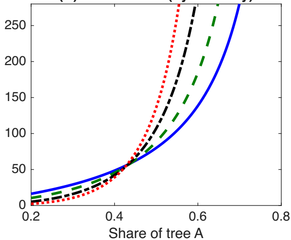
(D) CS of tree B (by maturity)
