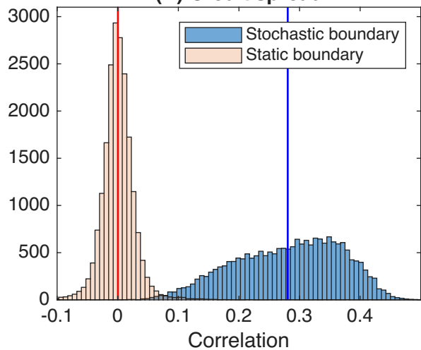
(D) Credit spread
