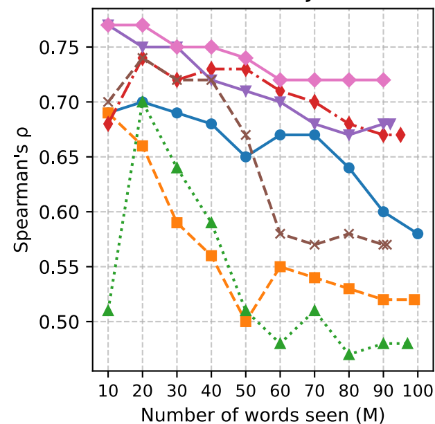
WUG ADJ
