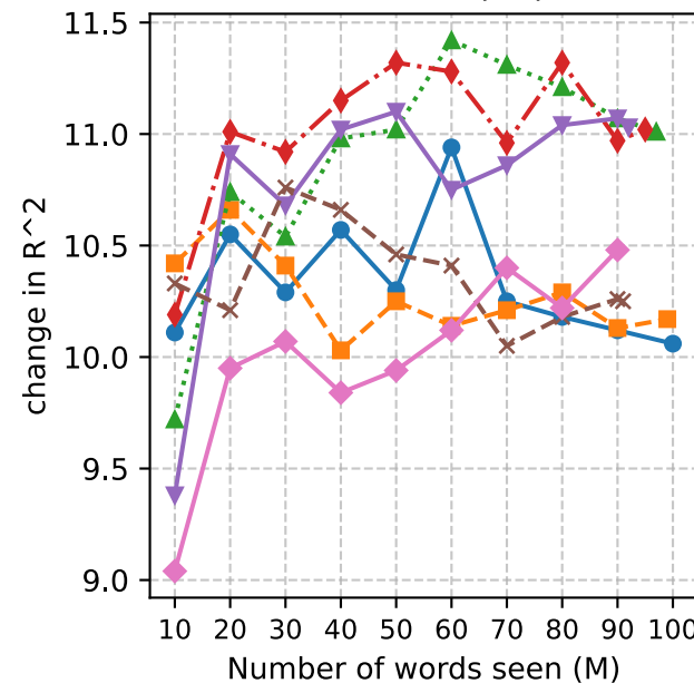
READING (ET)
