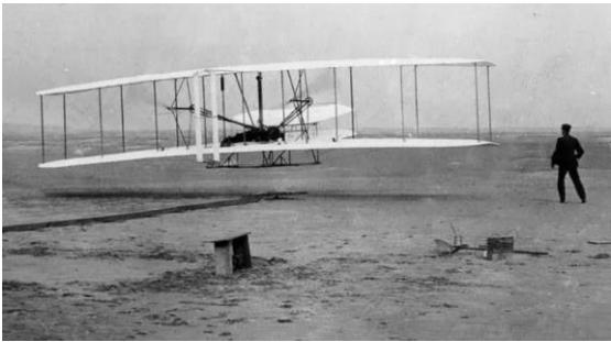
1903 年莱特兄弟的试验飞机
