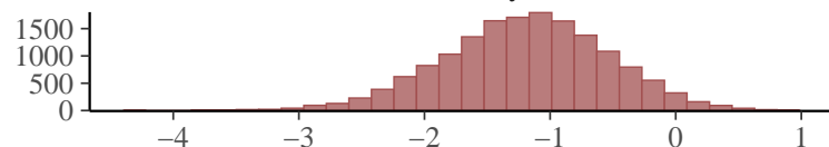
b_mudirhe_era_styledebated
