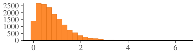
sd_lex__muprepdirhe_Intercept
