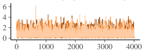
sd_lex__muprepdirhe_Intercept
