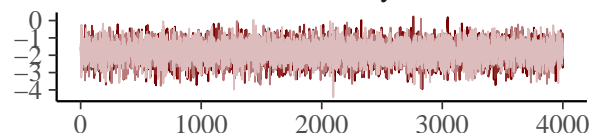
b_mudirhe_era_styleLBH
