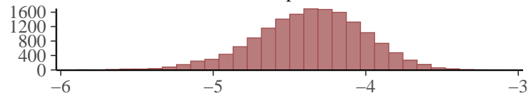
b_muvc_cmpl_animanim
