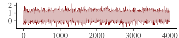
b_mvuc_verse_genrelist
