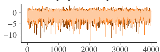
b_muprekdirhe_cmpl_detund
