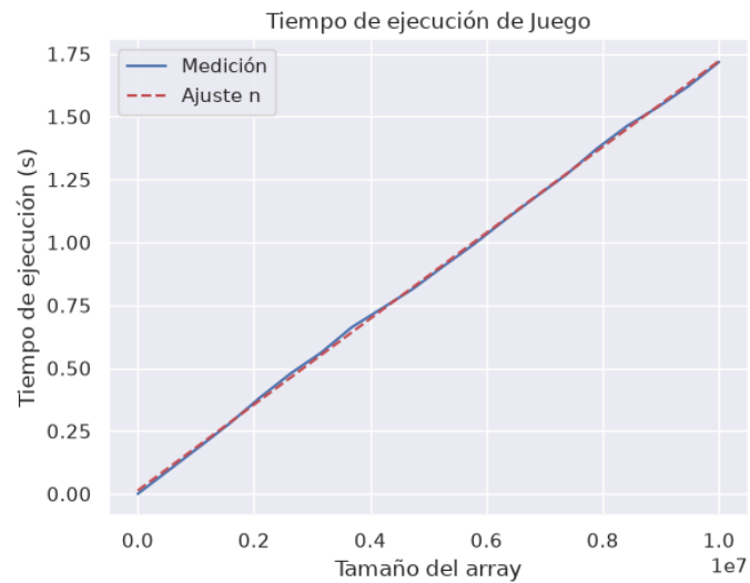
Figura 1: Tiempo de ejecución en función de la cantidad de elementos ( n ).
