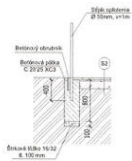
REZ A-A 1:50
