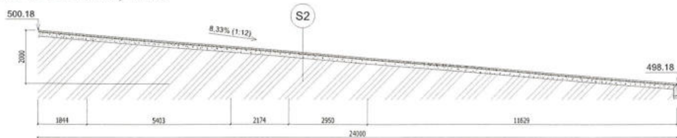
REZ B-B rozvinutý 1:100
