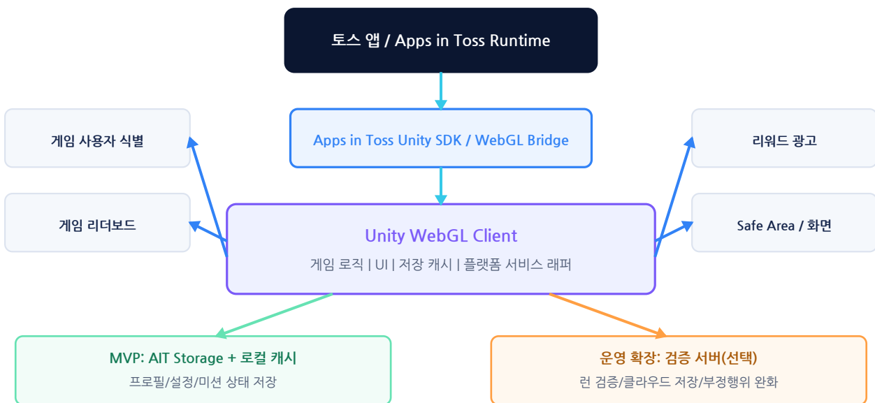
그림 4. Unity WebGL 클라이언트와 앱인토스 플랫폼 기능의 분리 구조
