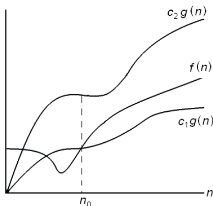
Obrázek 6.2: Znázornění funkce f(n) mezi c_1g(n) a c_2g(n) .
