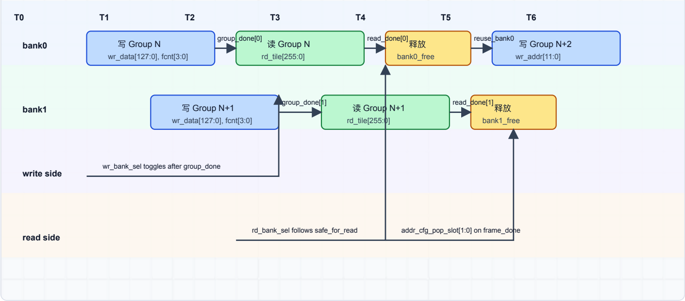
ENC ping-pong SRAM 时序图: 一次只讲 bank 占用和释放
