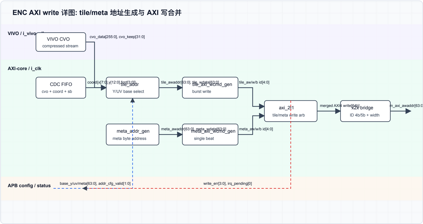
tile/meta write command、AXI merge/x2x 写出。
