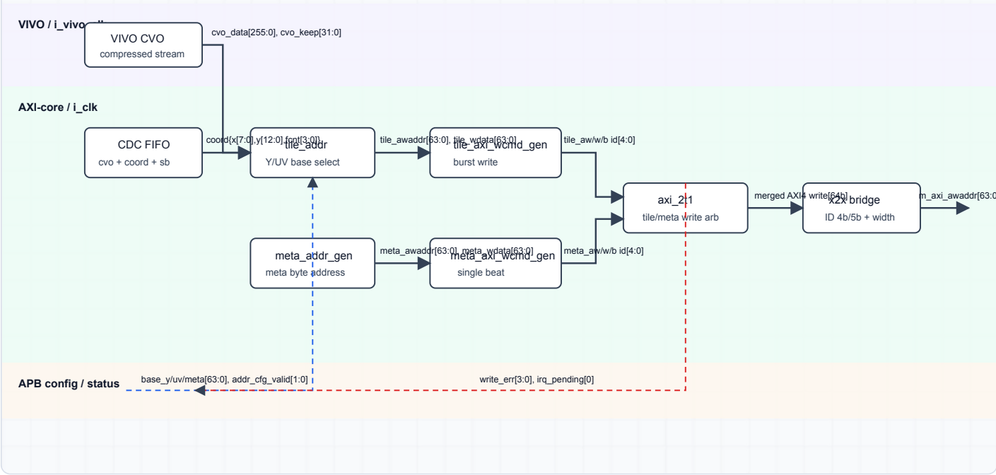
ENC AXI write 详图: tile/meta 地址生成与 AXI 写合并
